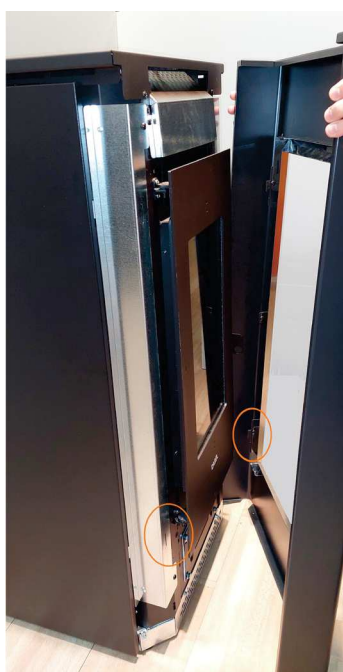
Fig. 30 - Desenganche del marco
