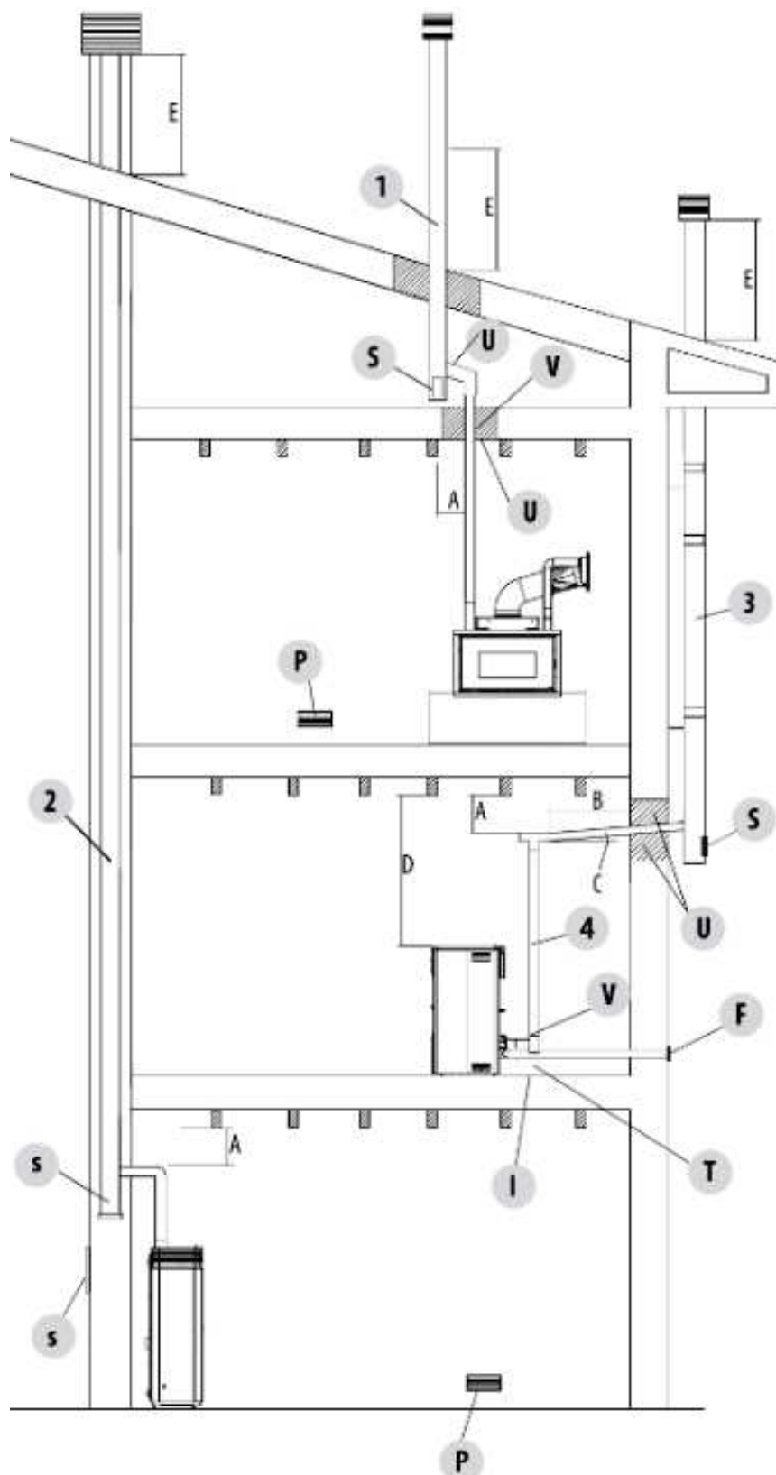
Fig. 13 - Sistema de evacuación de humos
