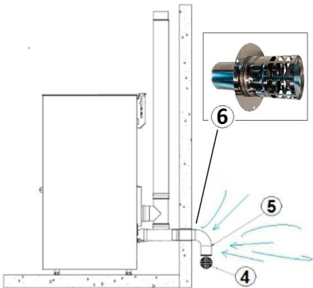
Fig. 8 - Toma de aire en caso de instalación estanca
