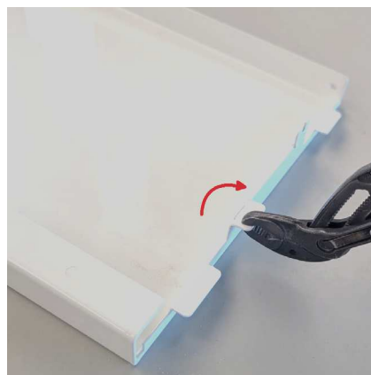
Fig. 38 - Pliegue las lengüetas hacia afuera
