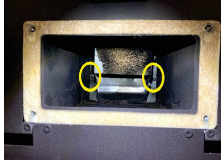
Fig. 129 - Desenrosque los tornillos
