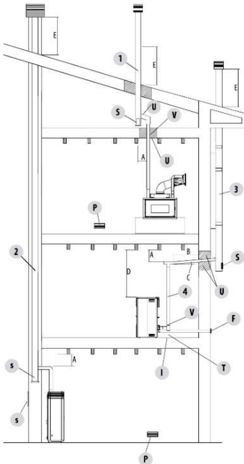
Fig. 10 - Sistema de evacuación de humos
