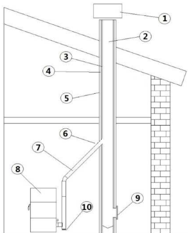
Fig. 2 - Componentes chimenea
