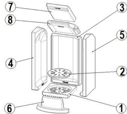
Nummerierung Keramott = Einbaureihenfolge!
