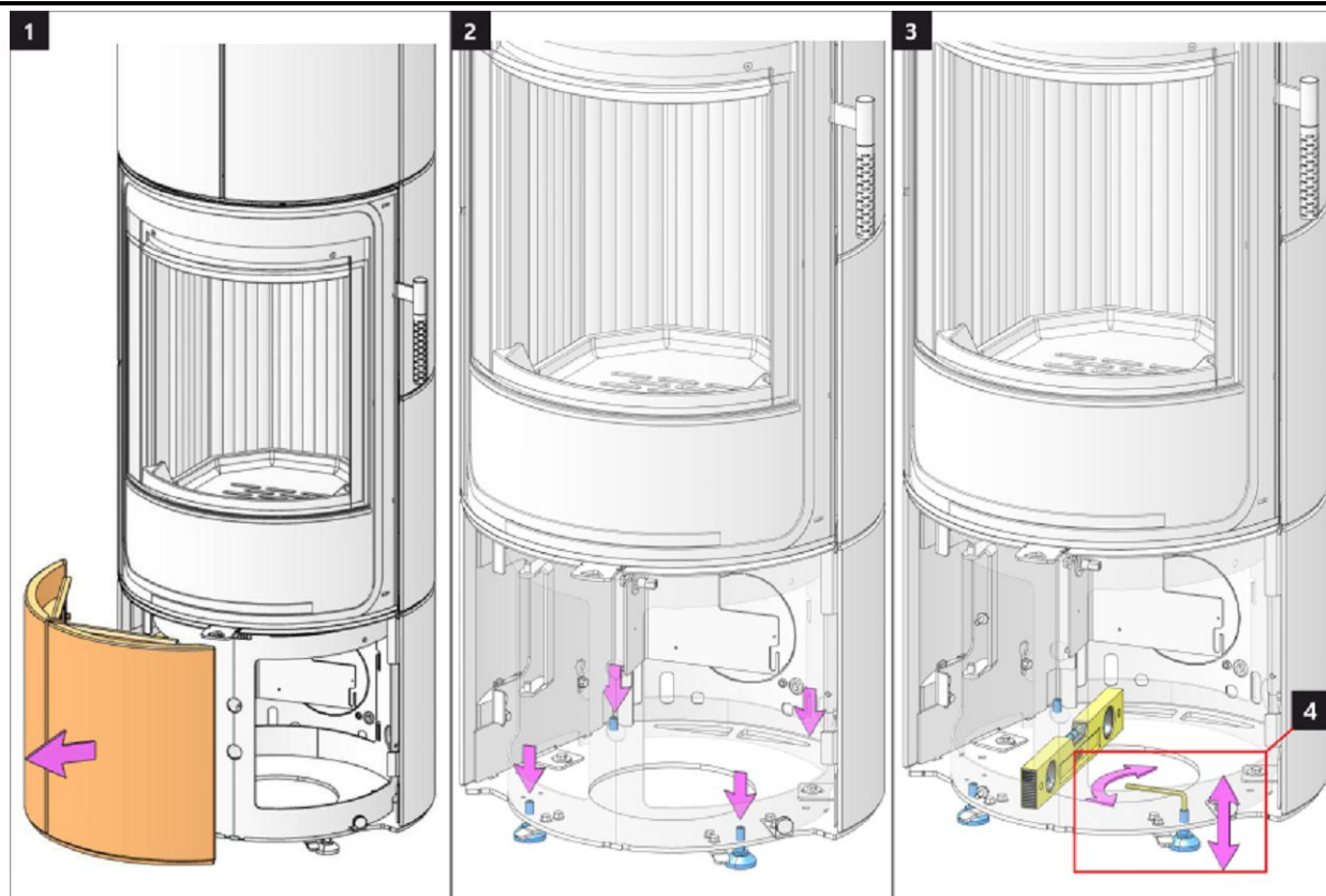
Product installation – Adjusting the feet 1 | Produktinstallation – Justierung der Füße 1 Installation du produit – Réglage des pieds 1 | Installazione del prodotto – Regolazione dei piedini 1
