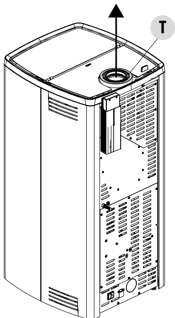
INSTALACIÓN TIPO «UP» SALIDA DE HUMOS DE PARED SIMPLE
