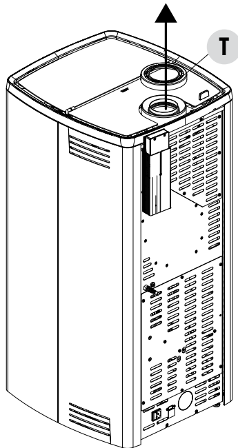
INSTALACIÓN TIPO «XUP» SALIDA DE HUMOS DE DOBLE PARED
