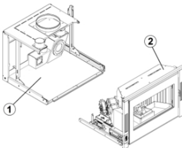
Fig. 25 - Estructura y cuerpo de la máquina
