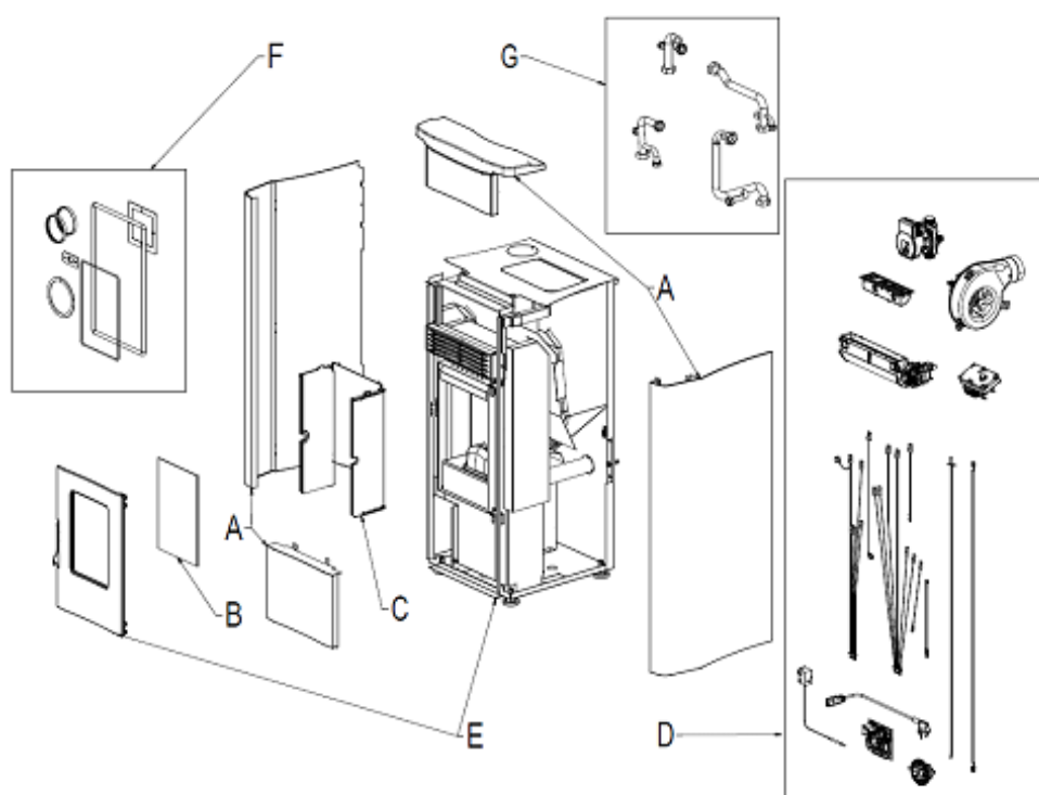
Fig. 1 - Dibujo explotado
