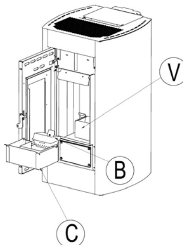
Fig. 33 - Limpieza
