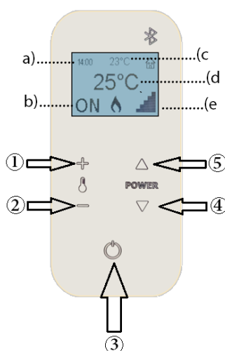
Fig. 29 - Mando a distancia con termostato
