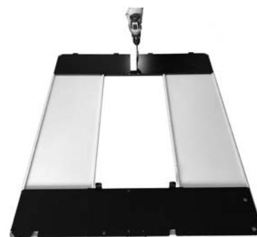
Fig. 38 - Fijación de los paneles
