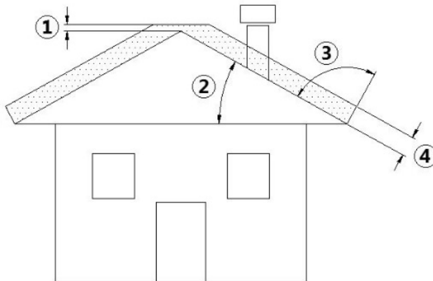
Fig. 3 - Techo inclinado
