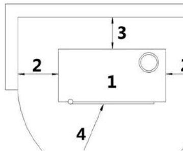
Fig. 22 - Instalación genérica con pedestal
