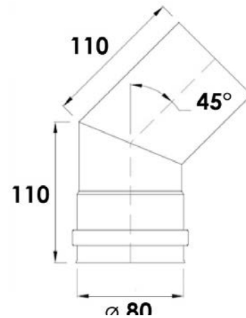
Fig. 21 - Curva a 45°
