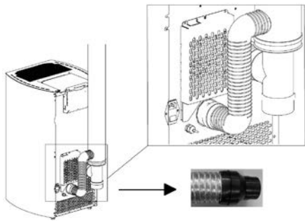
Fig. 13 - Tubo flexible
