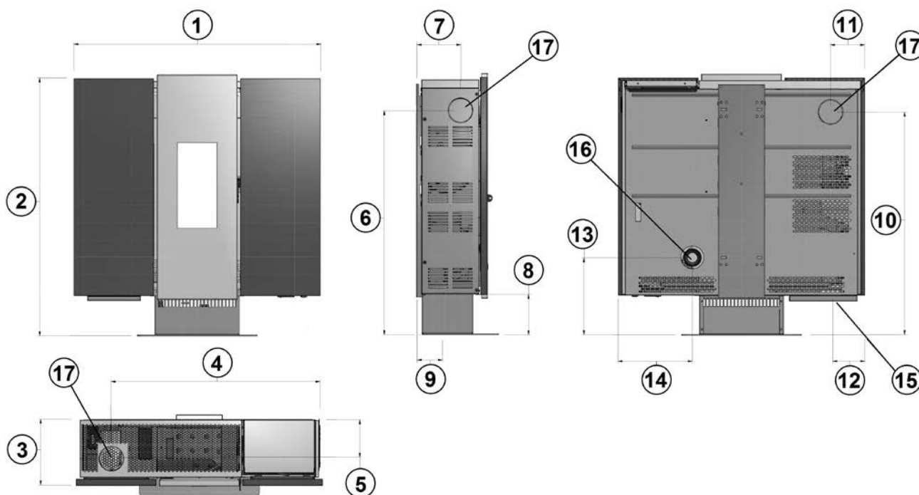
Fig. 16 - Dimensiones generales: Wall 3 Plus
