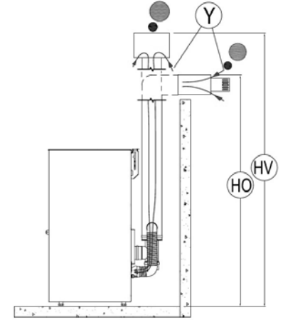
Fig. 15 - Conexiones del conducto de humos
