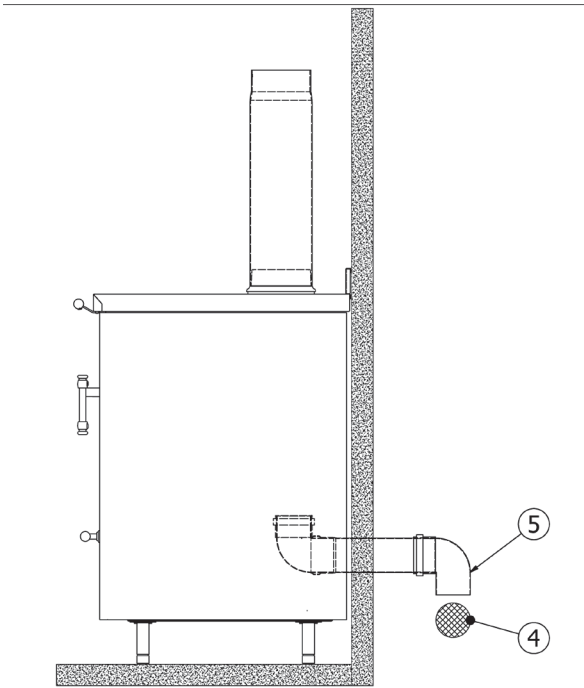
Fig. 7 - Afluencia del aire indirecta
