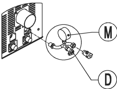
Fig. 64 - Terminal con grifo de carga (D) y manómetro (M)
