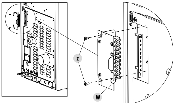
Fig. 75 - Conexiones
