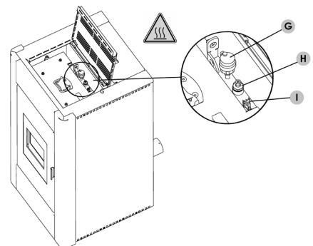
Fig. 66 - Válvula de purga manual (situada debajo de la parte superior)
