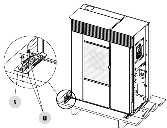
Fig. 3 - Eliminación de los estribos de fijación
