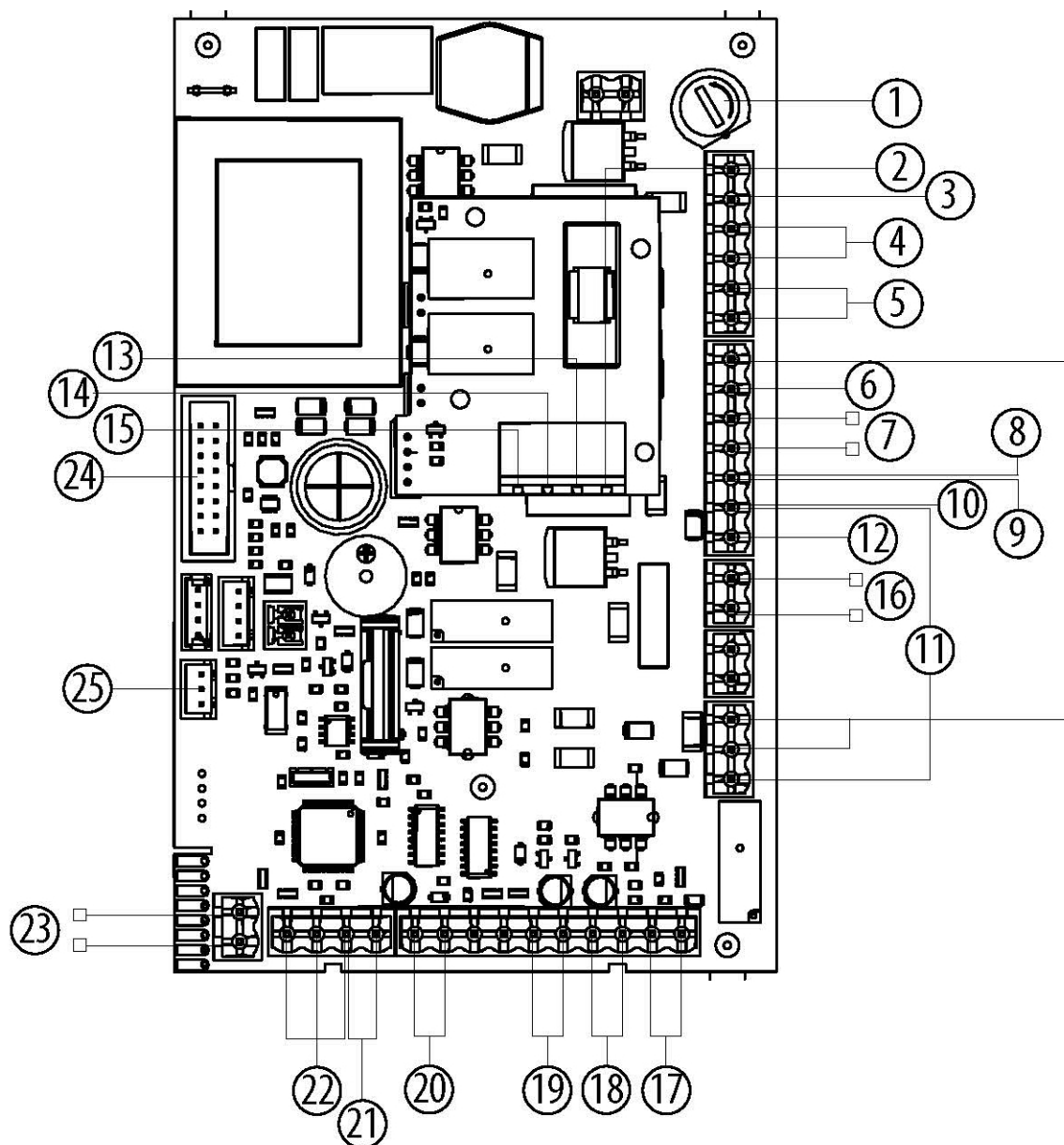
Fig. 100 - Tarjeta eléctrica
