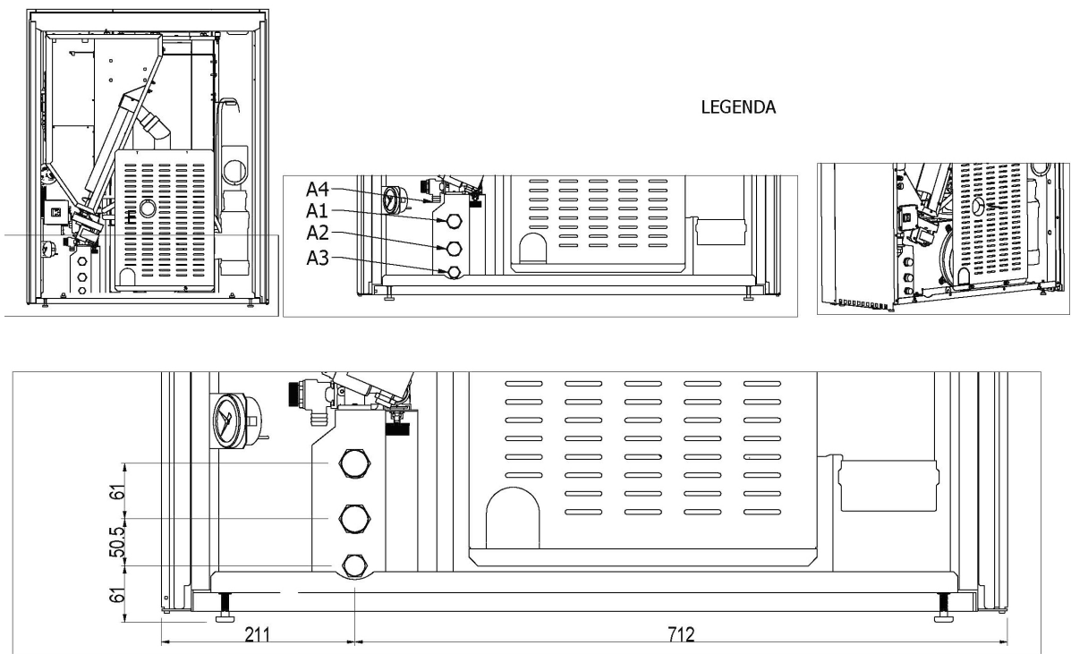
Fig. 62 - Esquema de conexión
