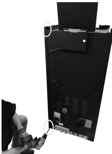
Fig. 52 - Fijación posterior del lateral
