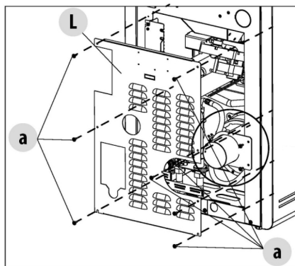
Fig. 52 - Panel posterior
