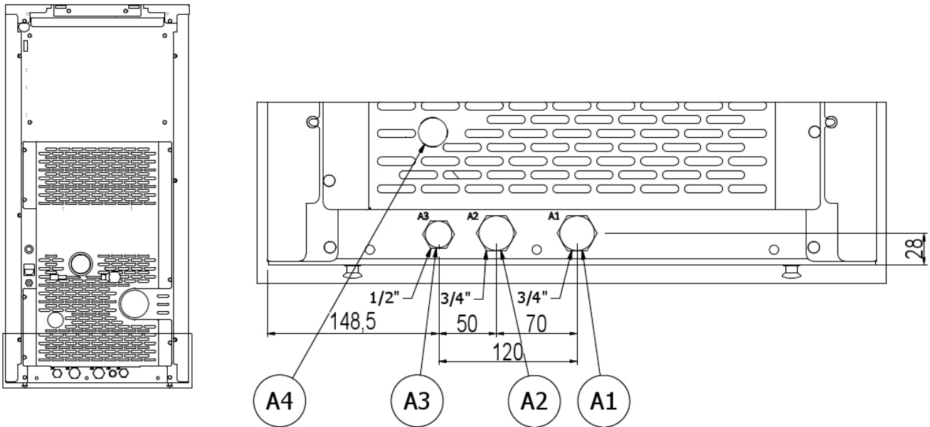
Fig. 36 - Esquema de conexión (sin ACS)
