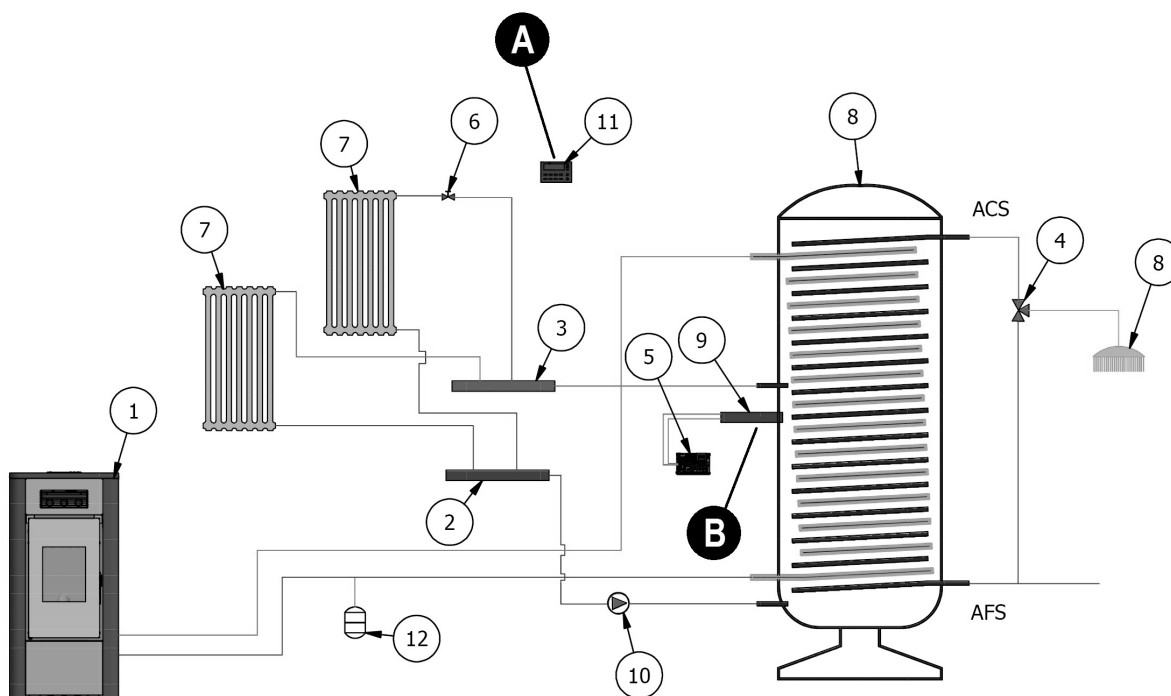
Fig. 46 - Configuración 5
