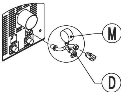
Fig. 39 - Terminal con grifo de carga (D) y manómetro (M)
