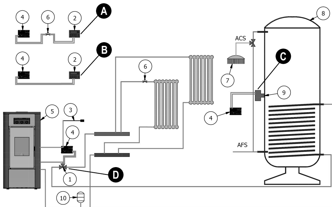
Fig. 43 - Configuración 2
