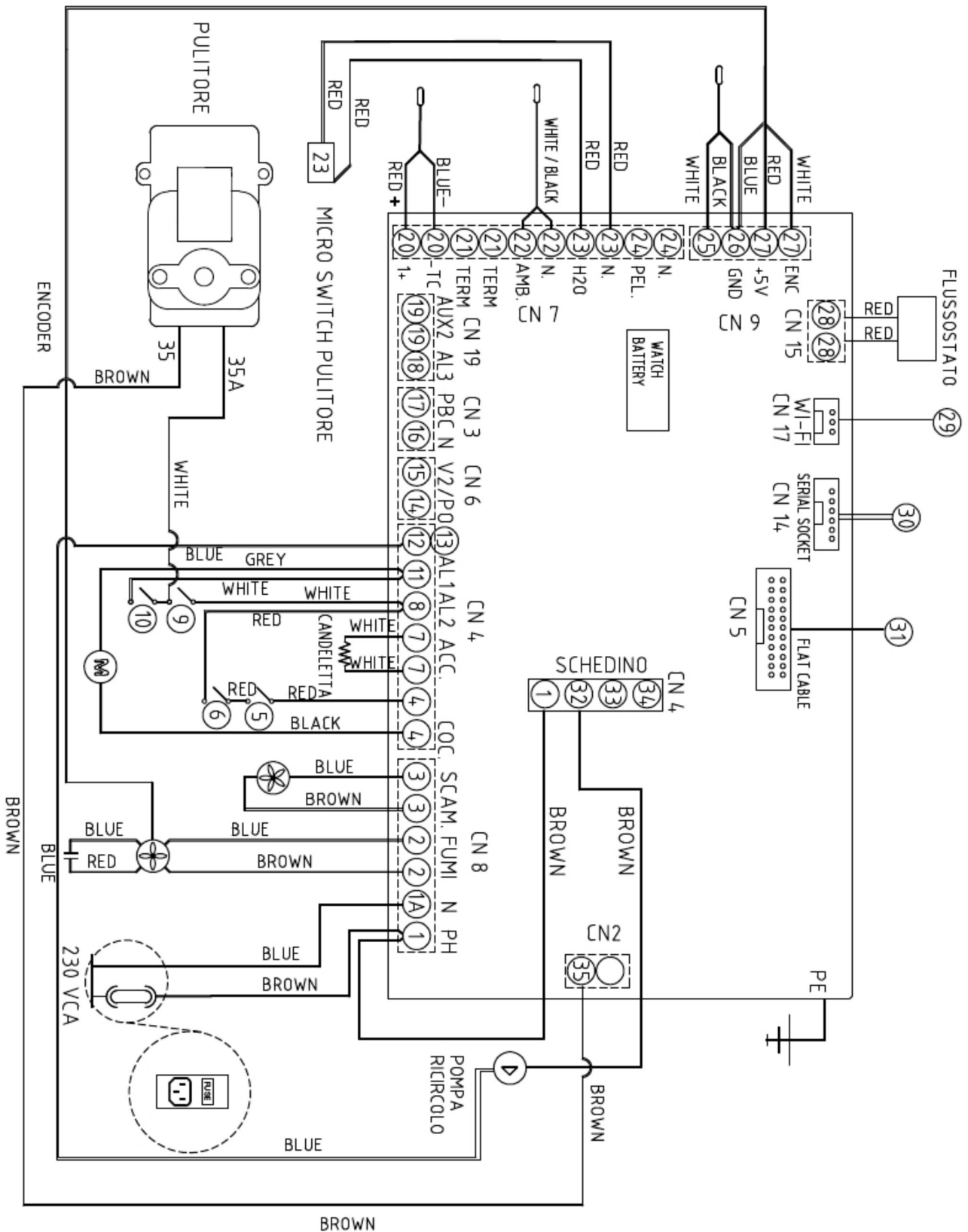
Fig. 69 - Tarjeta eléctrica senza ACS
