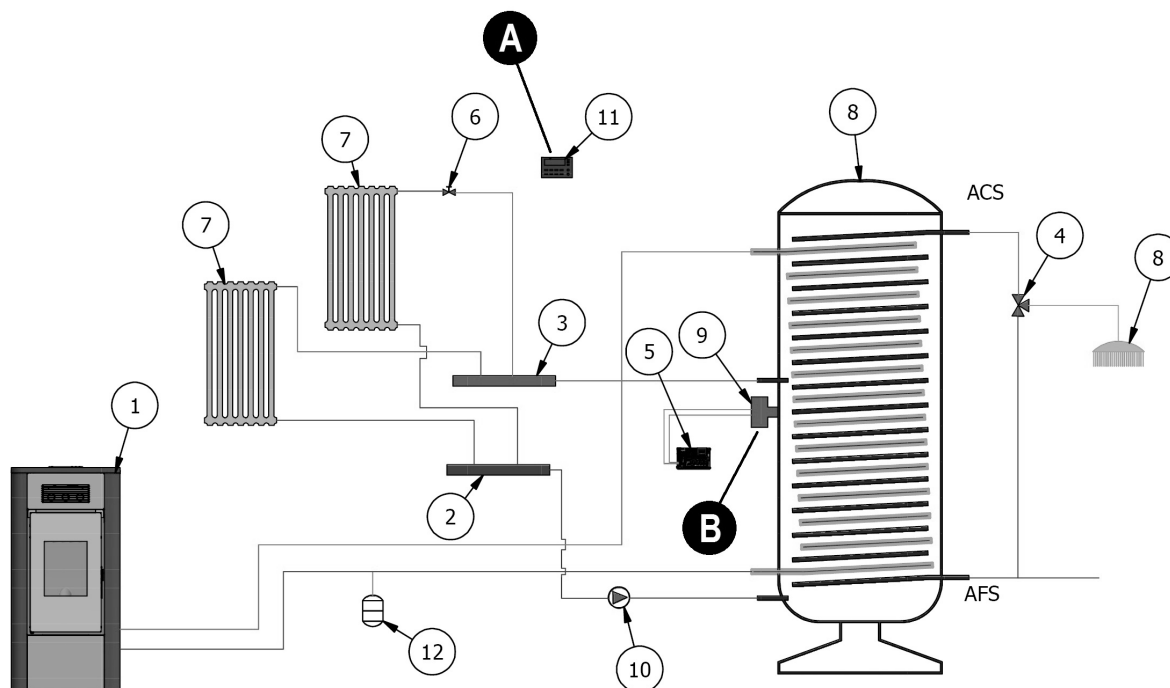
Fig. 45 - Configuración 4
