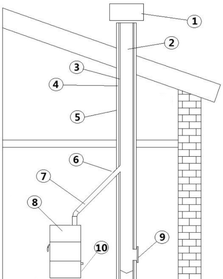
Fig. 5 - Componentes chimenea
