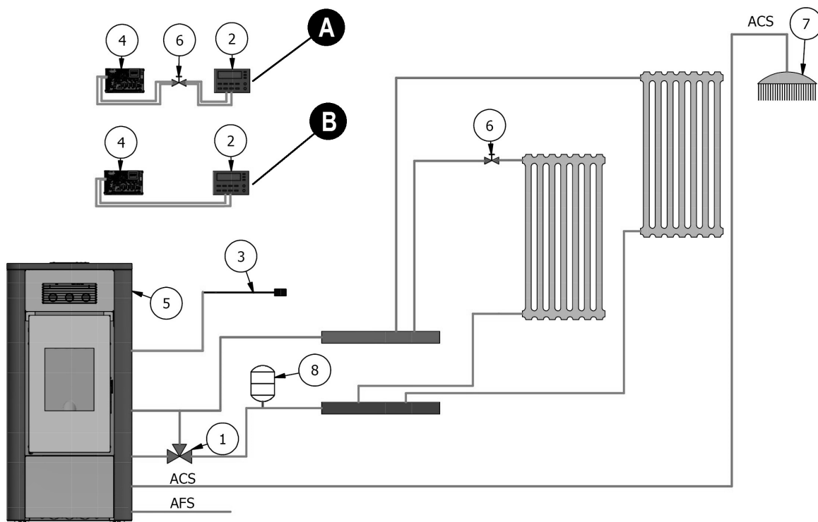
Fig. 42 - Configuración 2
