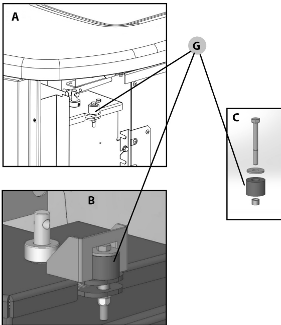
Fig. 67 - Goma
