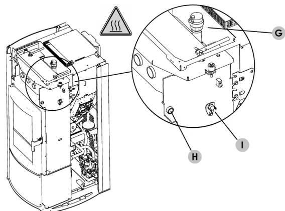
Fig. 40 - Válvula de purga manual (situada debajo de la parte superior) (Idro Prince 3 16-23-23 H2O, Aquos 3 16-23-23 H2O, Idron 16-22 Airtight, Hidrofire 22.8)
