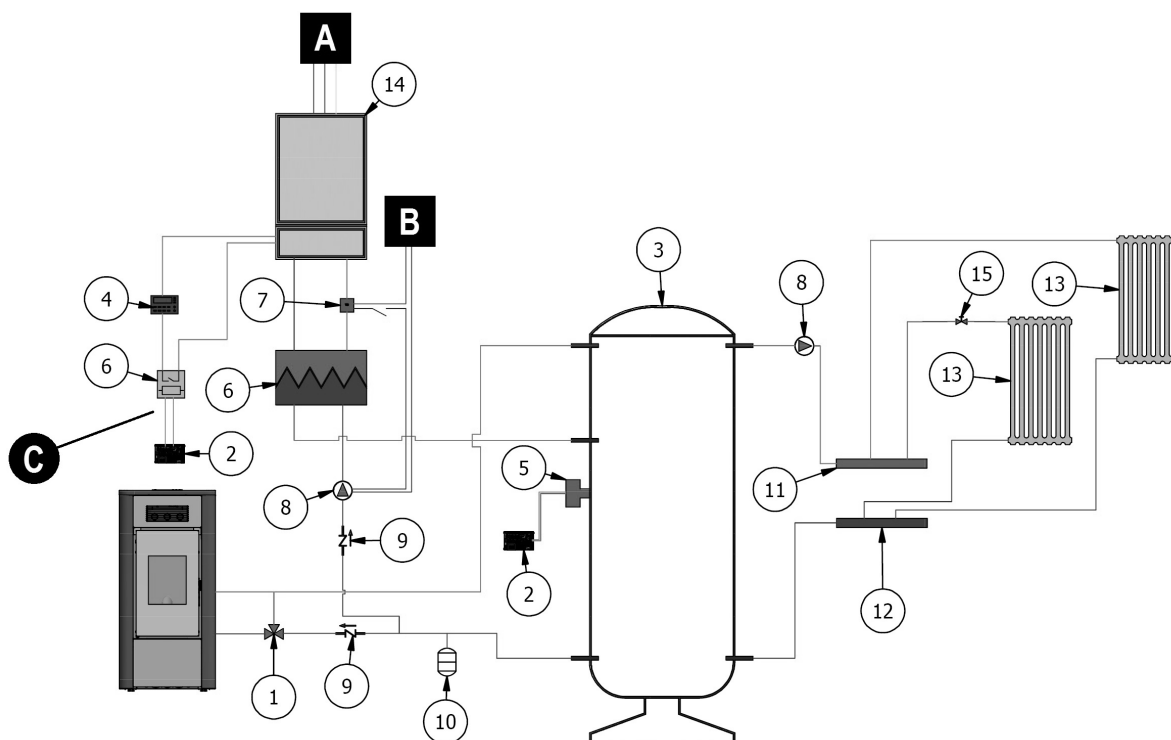
Fig. 47 - Configuración con calentador y caldera mural de auxilio
