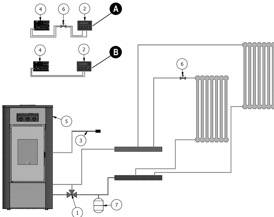
Fig. 41 - Configuración 1
