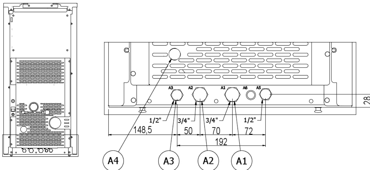
Fig. 37 - Esquema de conexión con ACS
