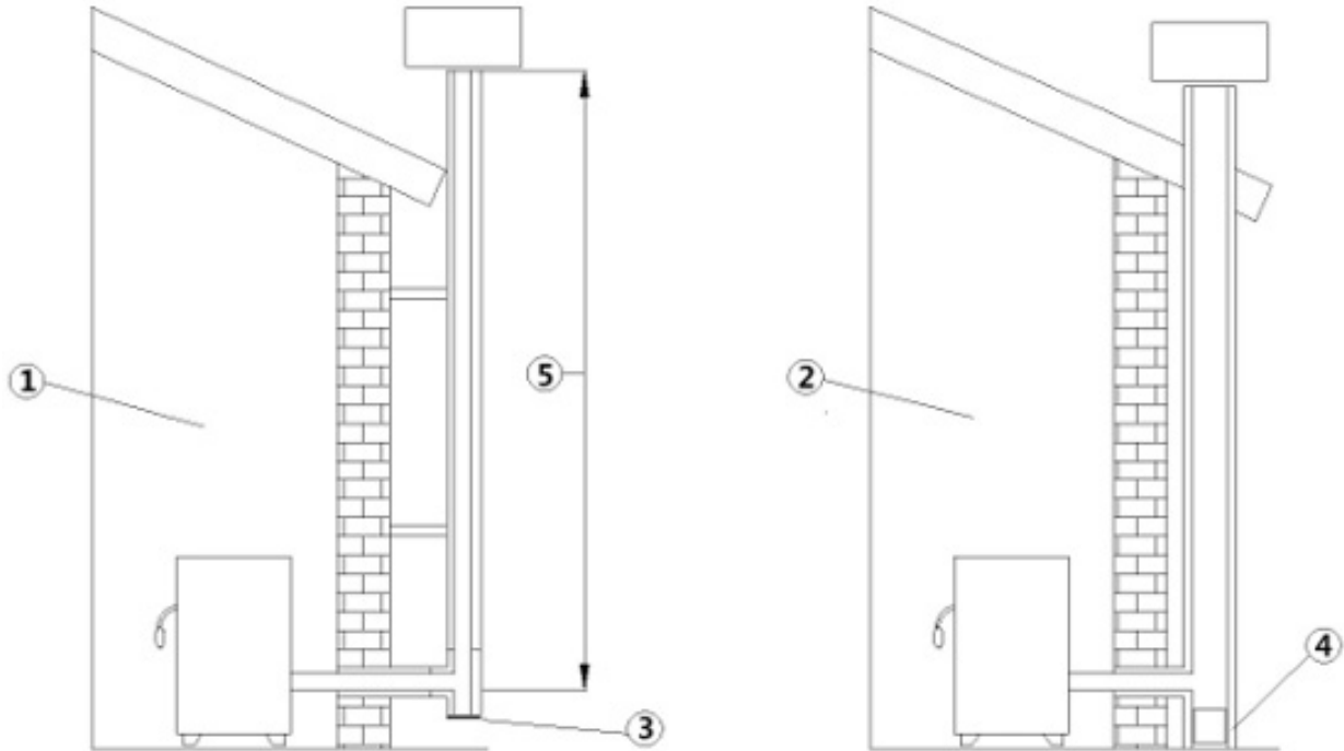
Fig. 8 - Conducto de chimenea
