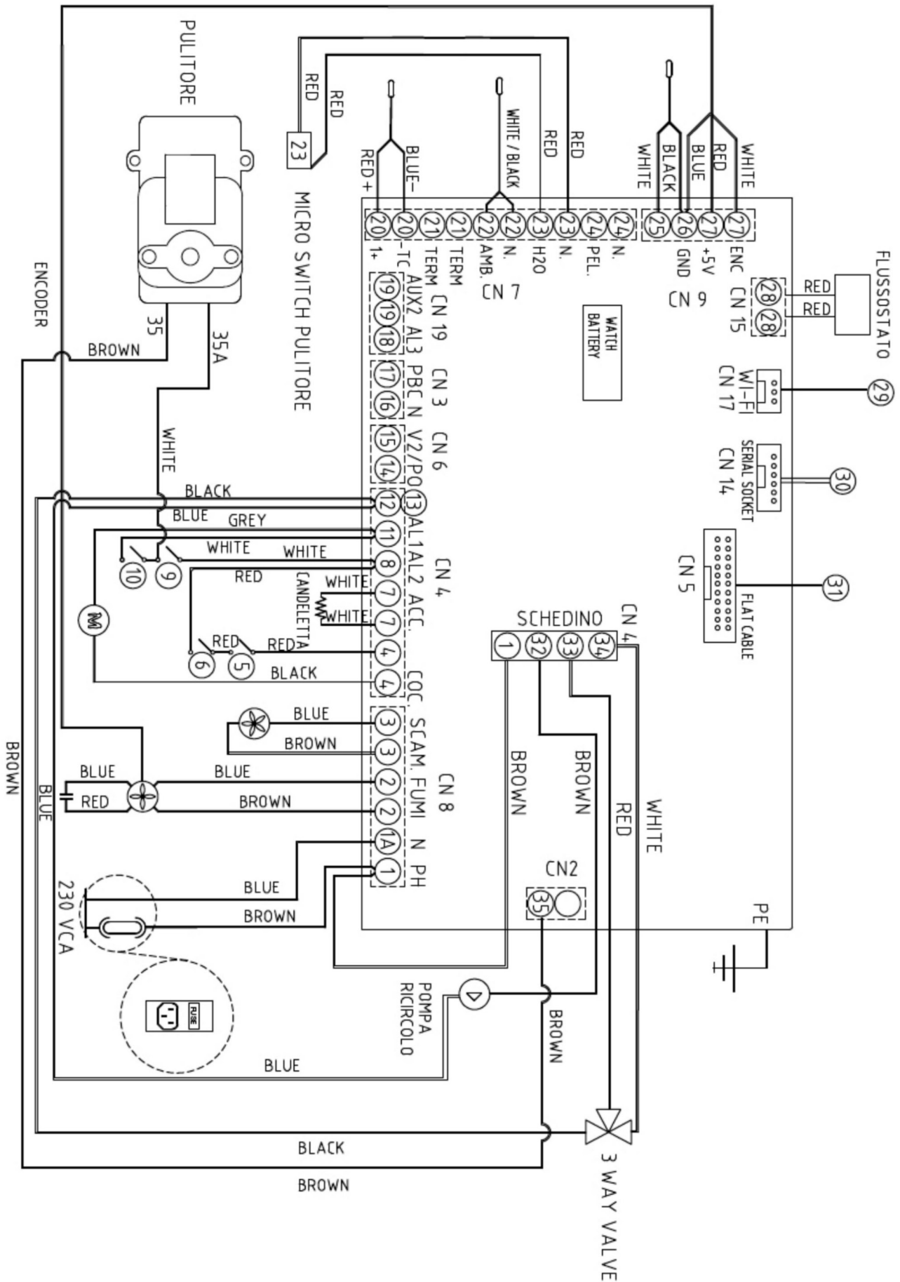
Fig. 70 - Tarjeta eléctrica con ACS
