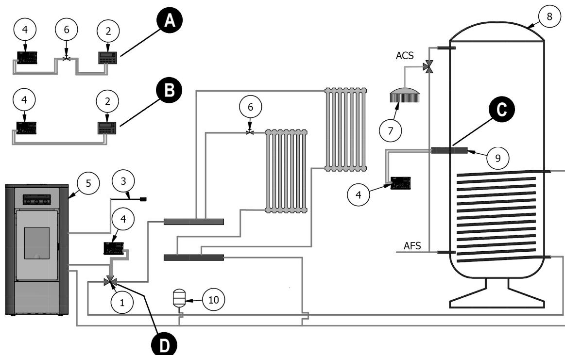
Fig. 44 - Configuración 3
