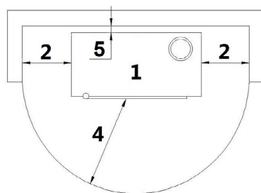
Fig. 77 - Instalación en pared
