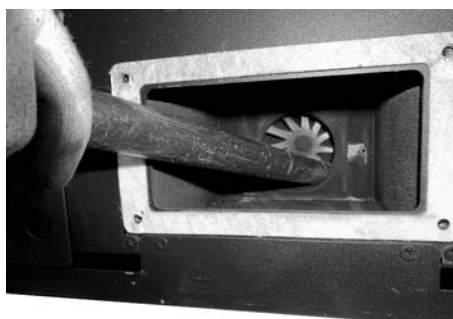
Fig. 126 - Aspire las cenizas
