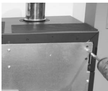
Fig. 48 - Desatornillar 1
