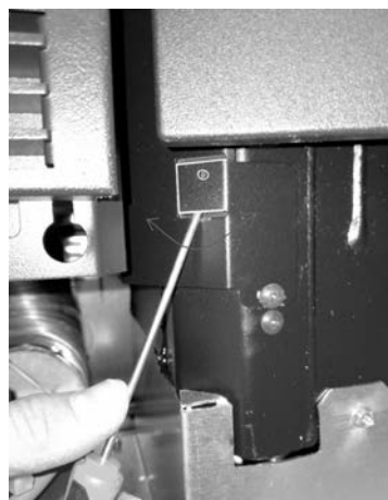
Fig. 46 - Levantar aletas 2
