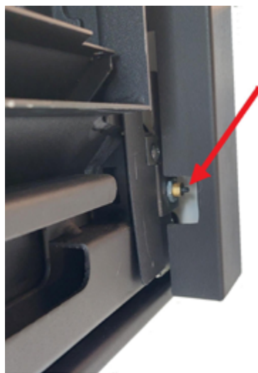
Fig. 41 - El reinicio manual se encuentra en la parte frontal, lado derecho (ZEFIRO 2026)
