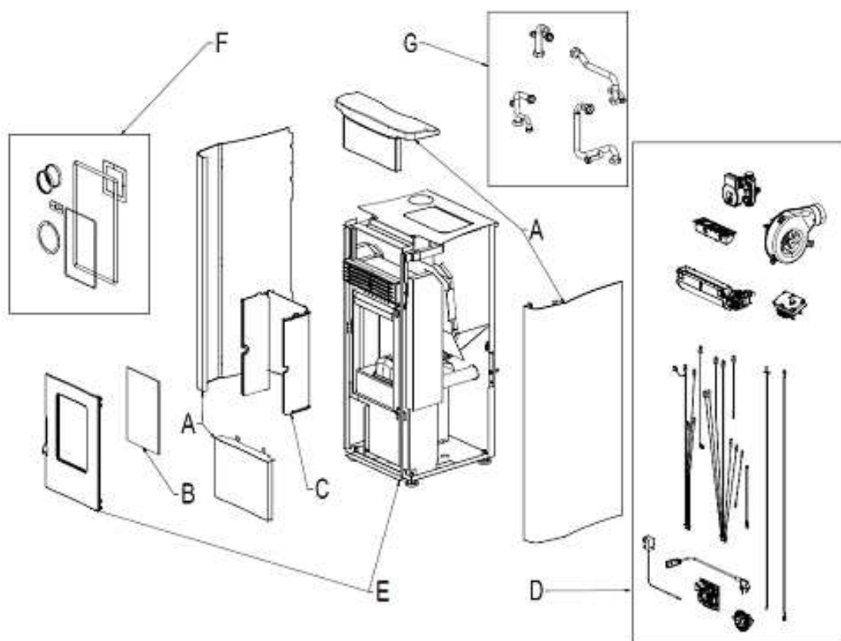
Fig. 1 - Dibujo explotado
