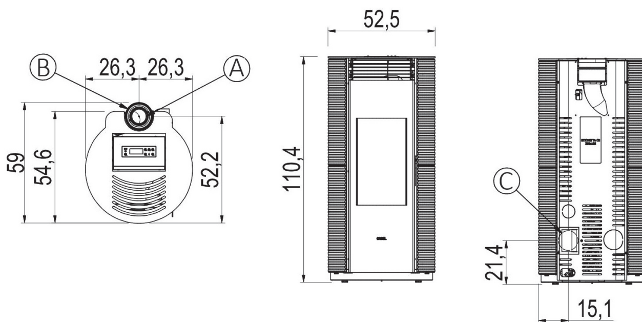
Fig. 15 - SPIN PLUS 9 UPTW K1 - SPIN PLUS 9 UP-TWIN T1 - SPIN PLUS 7 UP-TWIN T1
