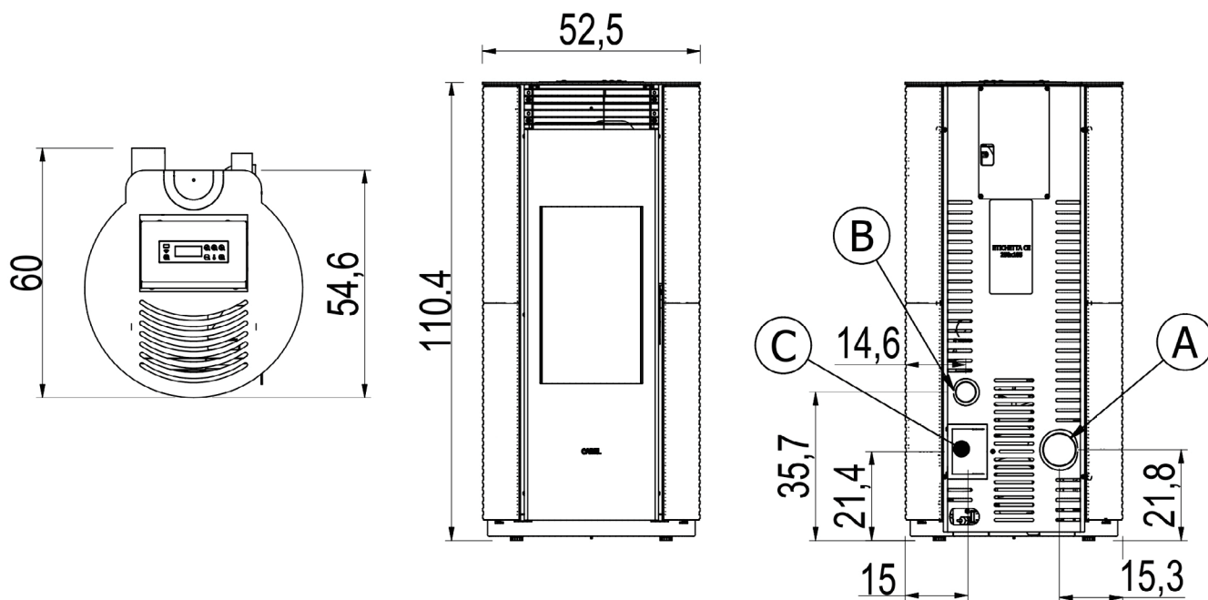
Fig. 16 - SPIN PLUS 9 T1 - SPIN PLUS 9 K1
