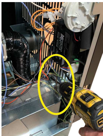
Fig. 54 - Bloqueo del tubo flexible
