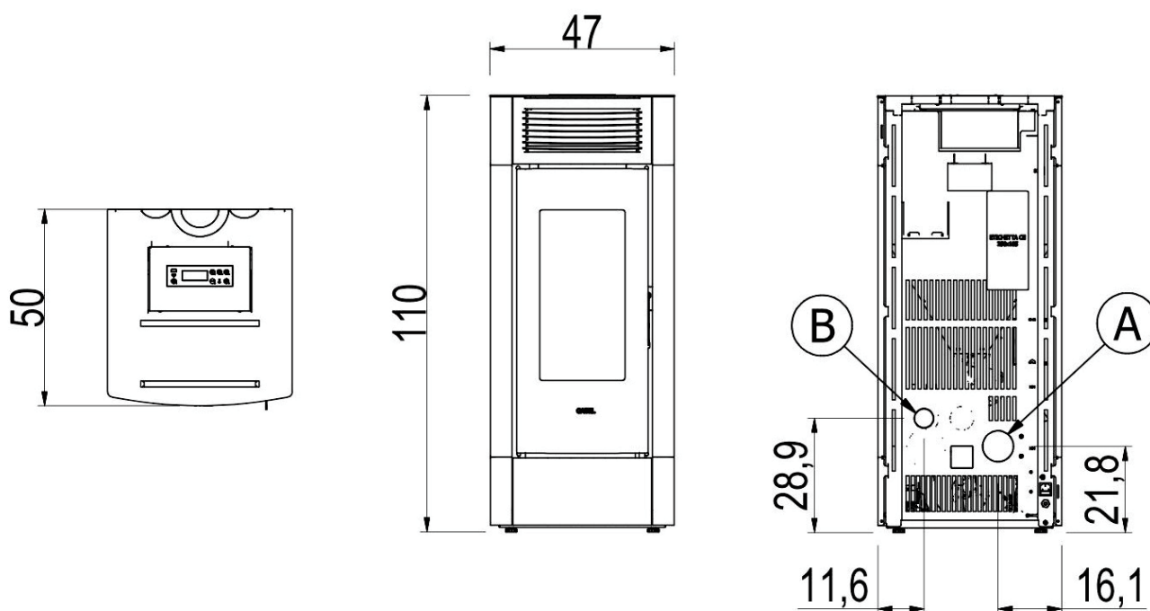
Fig. 19 - CRISTAL 9 AIR T1 - CRISTAL 9 AIRTECH T1 - CRISTAL 9 K1
