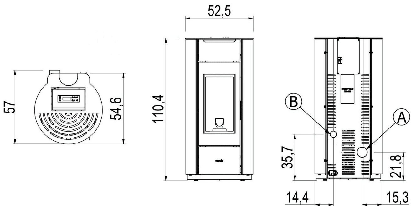
Fig. 17 - EOS 8 T1 - EOS 8 K1
