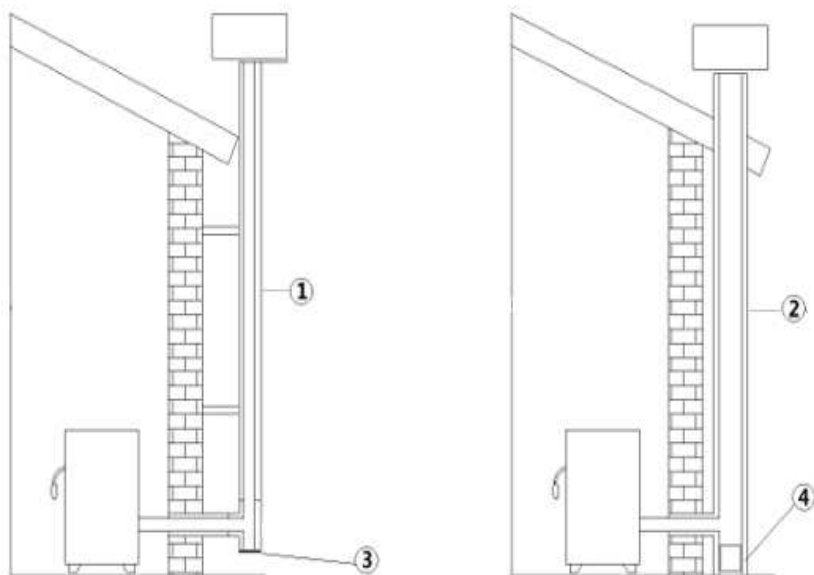
Fig. 5 - Conducto de chimenea
