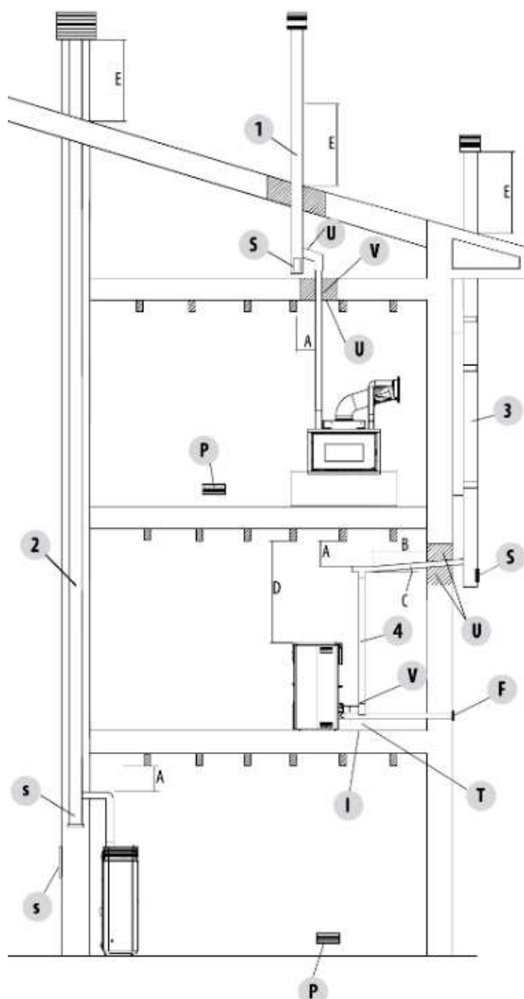
Fig. 13 - Sistema de evacuación de humos
