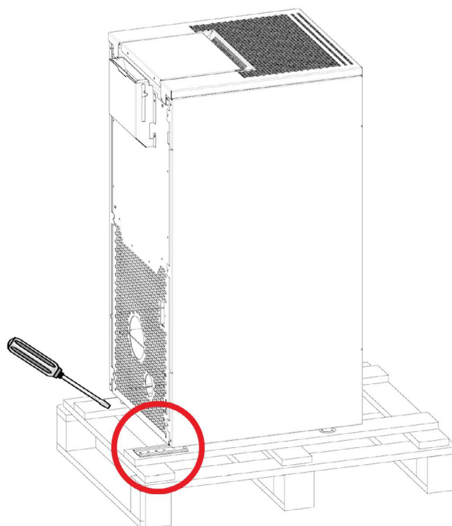
Fig. 1 - Extracción de las abrazaderas
