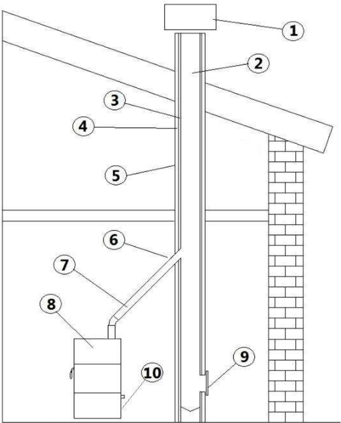
Fig. 2 - Componentes chimenea
