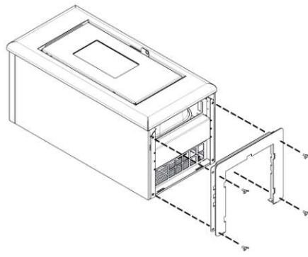
Fig. 52 - Montaje del pedestal
