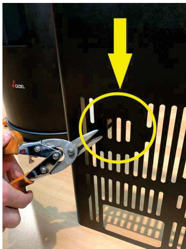
Fig. 63 - Romper el anillo
