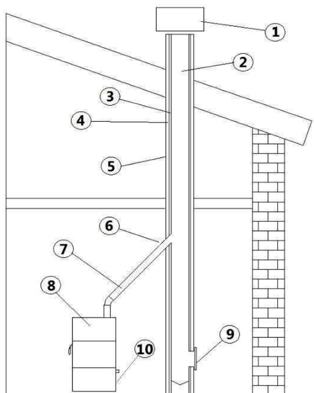
Fig. 2 - Componentes chimenea
