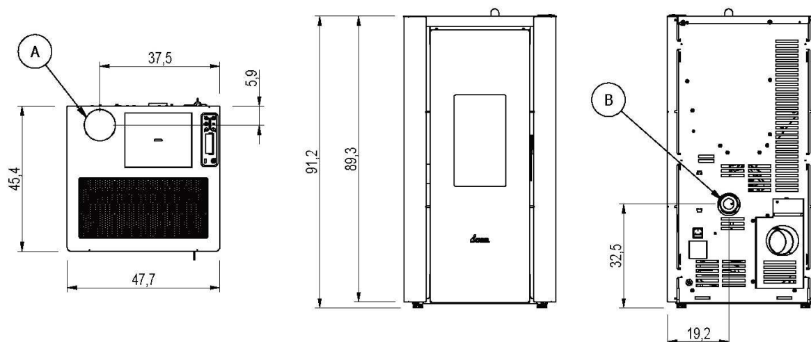
Fig. 28 - Dimensiones generales: CRISTAL 7UP
