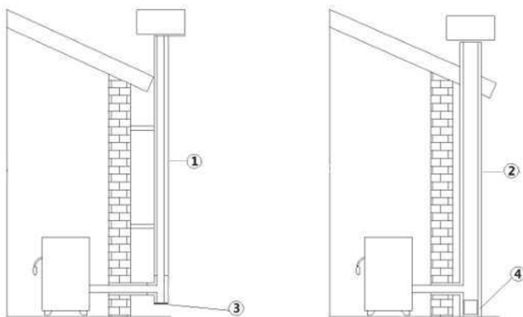
Fig. 5 - Conducto de chimenea
