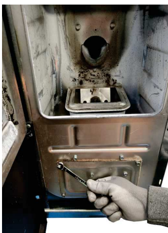
Fig. 79 - Quite los tornillos
