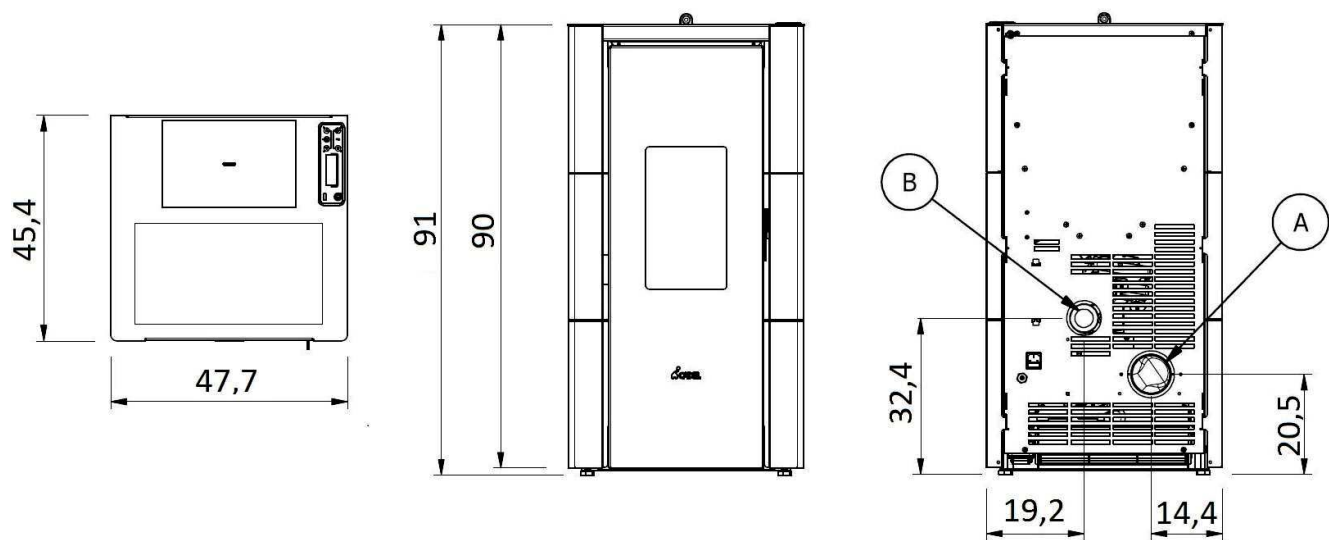
Fig. 16 - Dimensiones generales: CRISTAL 7 -
