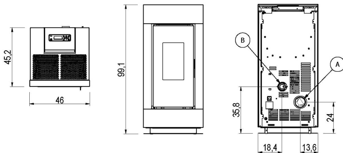
Fig. 23 - Dimensiones generales: LEYENDA
