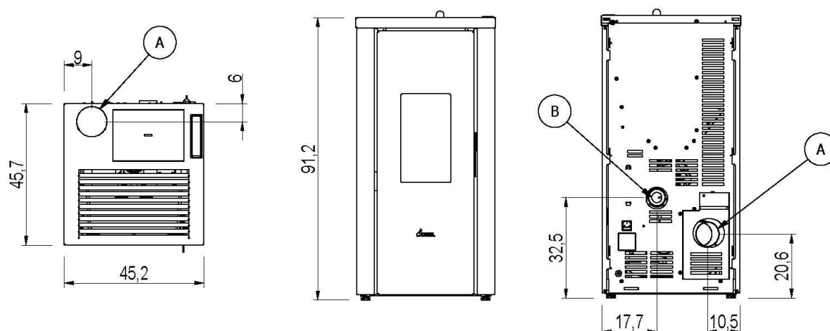
Fig. 27 - Dimensiones generales: --
