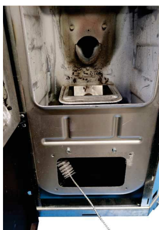
Fig. 81 - Limpie con una escobilla
