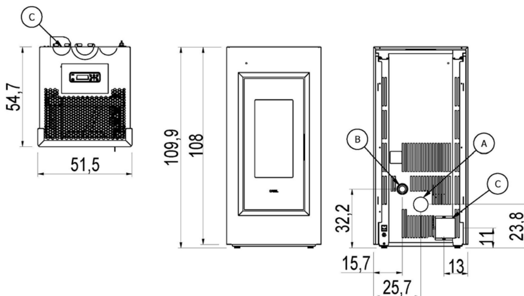
Fig. 14 - Dimensiones generales: Prince 11 - Prince Plus 11
