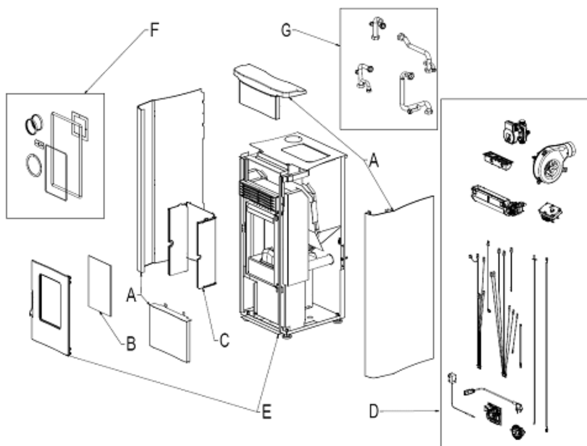
Fig. 1 - Dibujo explotado
