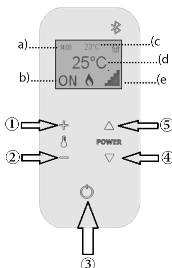
Fig. 29 - Mando a distancia con termostato
