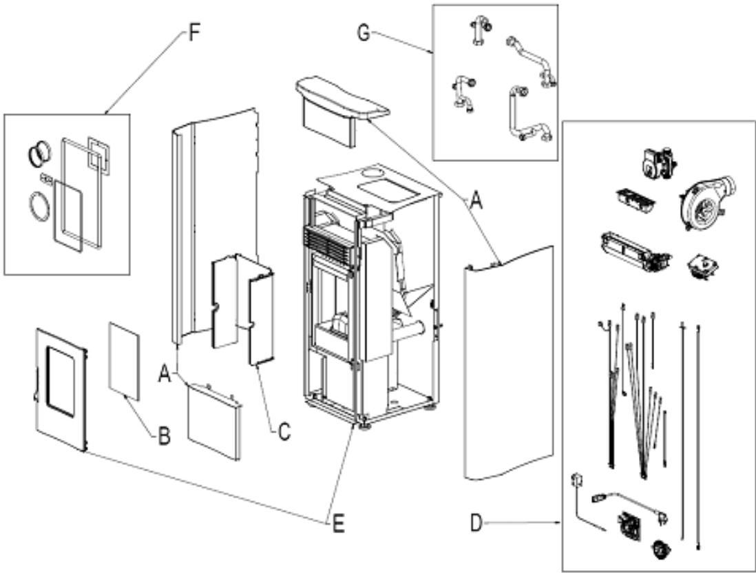
Fig. 1 - Dibujo explotado
