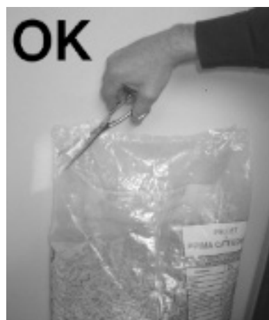
Fig. 23 - Abertura correcta del saco del pellets
