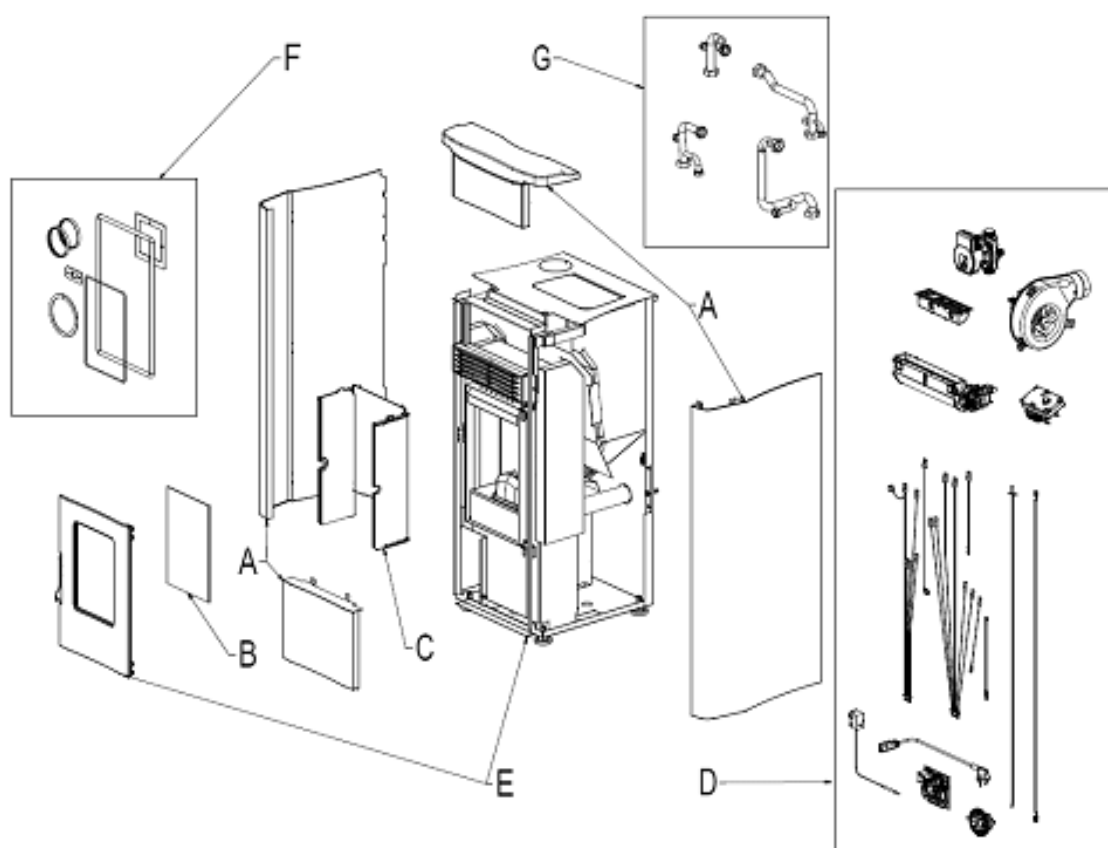
Fig. 1 - Dibujo explotado
