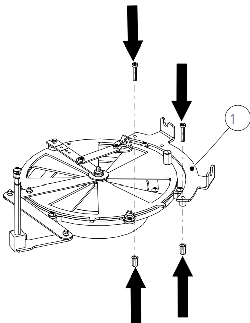
Abb. 11: Montageset montieren
