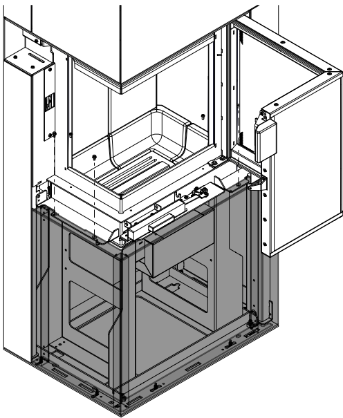
Fig. 27: Fixer l'habillage inférieur
