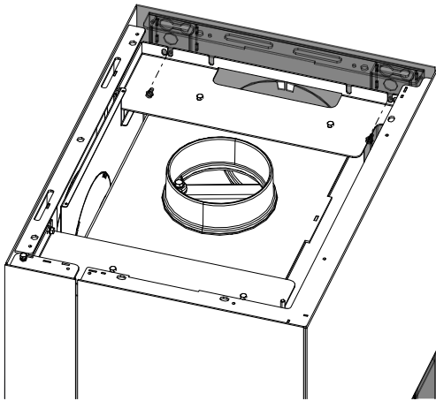
Abb. 31: Seitenwand demontieren
