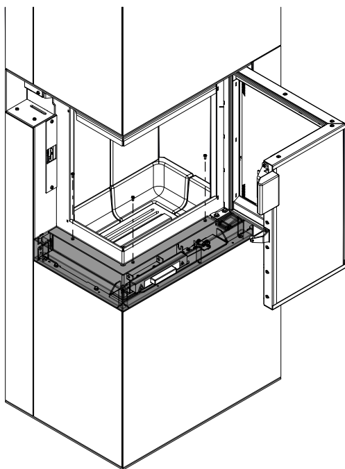
Fig. 28: Fixer le cache
