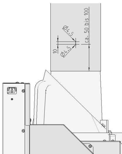
Fig. 5: Schéma de perçage pour conduit de fumée
