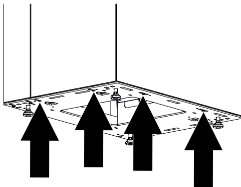
Abb. 29: Blende von unten festschrauben
