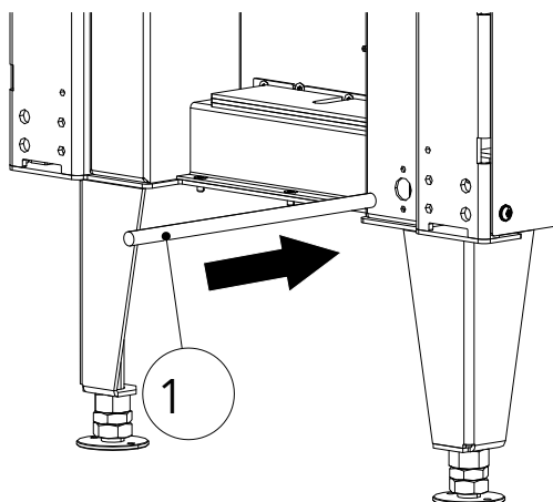
Fig. 13: Enfiler le câble Bowden
