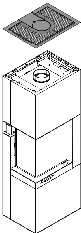
Fig. 35: Montaggio del coperchio
