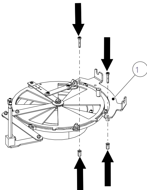
Fig. 11: Installazione del kit di montaggio
