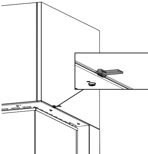
Abb. 22: Spaltmaß einhalten
