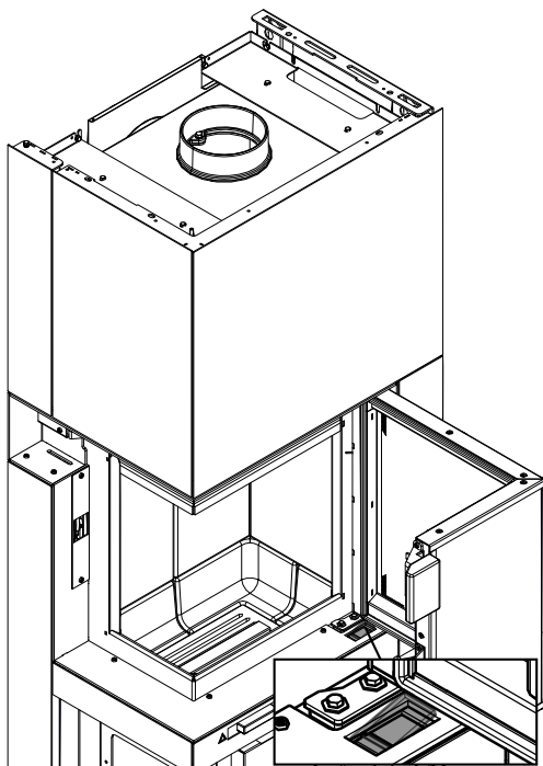
Fig. 25: Fixer la porte
