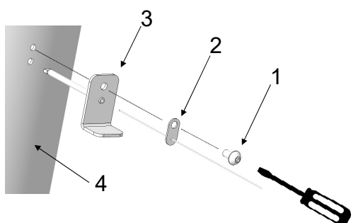
Fig. 6: Montaggio del sensore di temperatura
