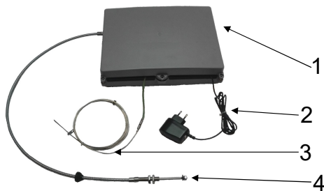
Abb. 1: Steuerungseinheit
