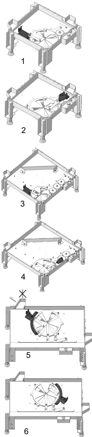
Abb. 7: Einbau K Ecke links rechts
