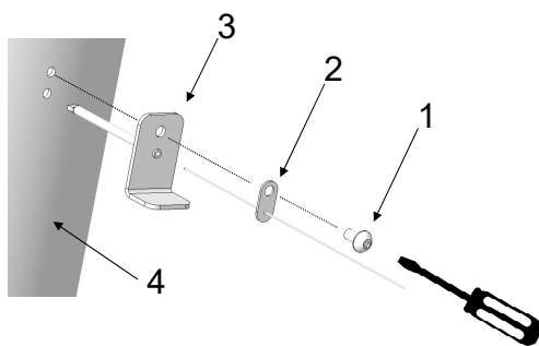
Abb. 6: Temperatur-Sensor montieren
