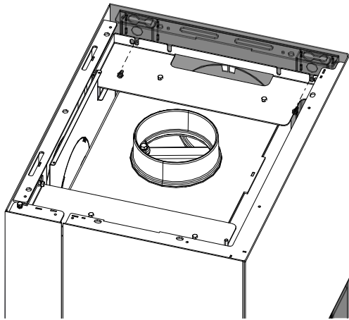
Abb. 33: Seitenwand montieren
