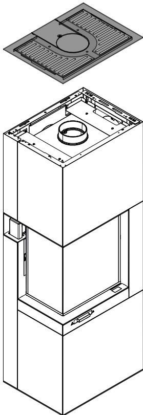
Abb. 35: Deckel montieren
