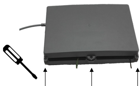
Fig. 17: Débrancher le bloc d'alimentation
