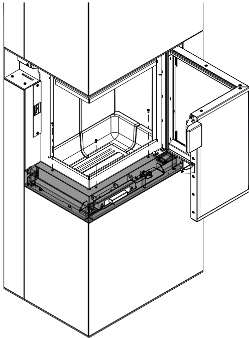
Abb. 28: Blende befestigen
