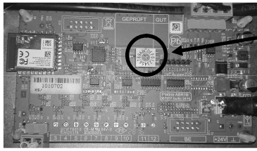
Fig. 18: Selezione del programma
