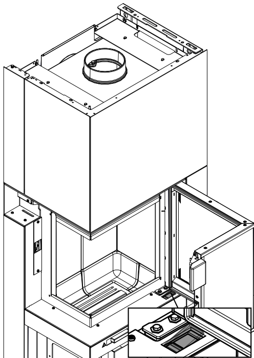
Fig. 25: Fissare la porta
