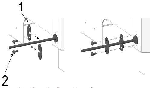
Fig. 16: Flangia Cavo Bowden
