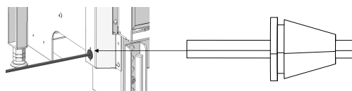
Fig. 15: Enclencher le bouchon en caoutchouc
