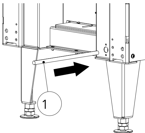
Fig. 13: Inserimento del cavo Bowden
