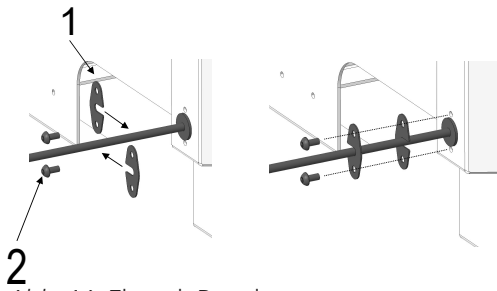
Abb. 16: Flansch Bowdenzug
