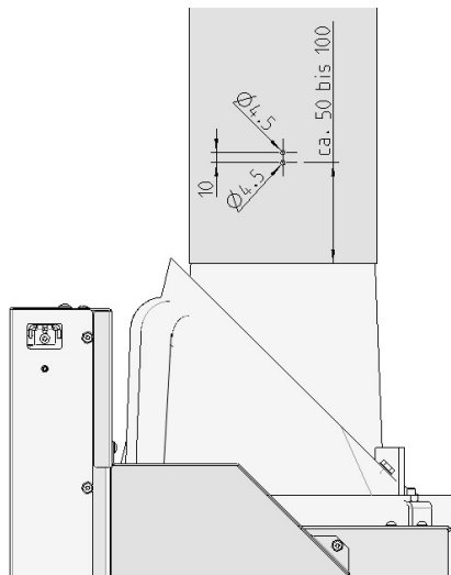
Abb. 5: Bohrschema-Rauchrohr
