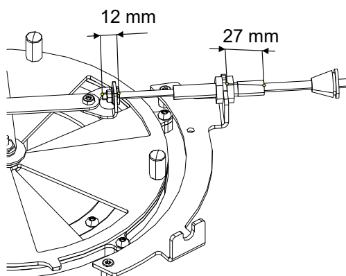
Fig. 14: Collegamento del cavo Bowden
