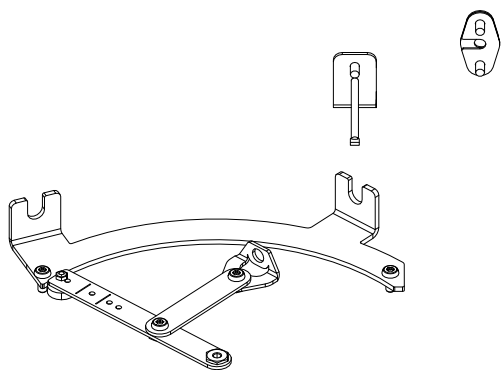
Fig. 3: Kit de montage 363004
