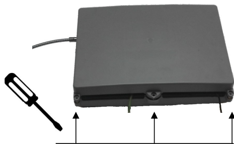
Abb. 17: Netzteil ausstecken
