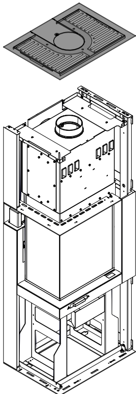
Fig. 19: Enlever le couvercle
