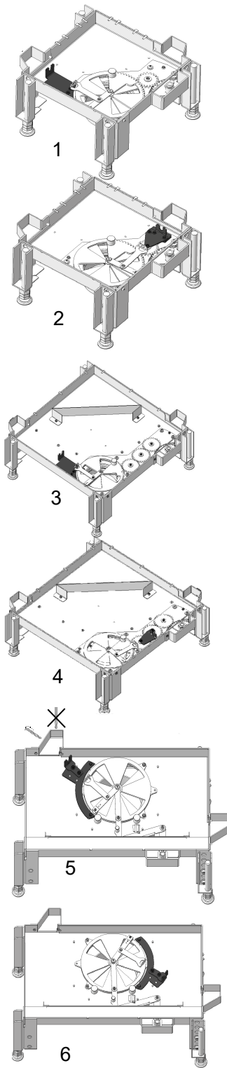
Fig. 7: Montaggio angolo K sx e dx
