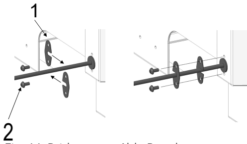
Fig. 16: Brides pour câble Bowden
