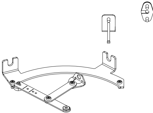
Fig. 3: Kit di montaggio 363004
