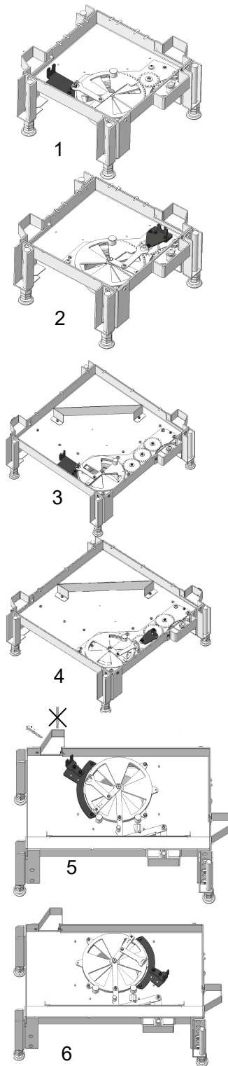
Fig. 7: Installation K en angle à gauche à droite
