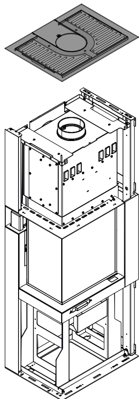
Fig. 19: Rimuovere il coperchio
