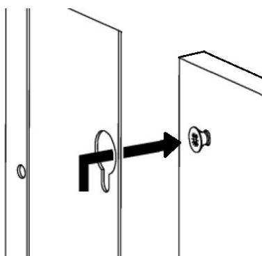
Fig. 25 - Sistema de acoplamiento
