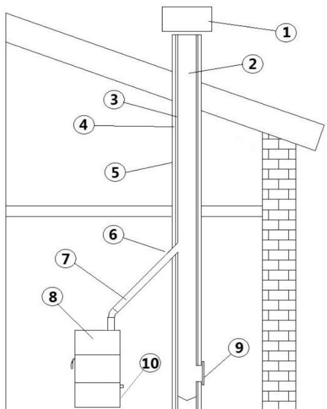
Fig. 2 - Componentes chimenea
