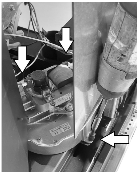
Fig. 100 - Quite los tornillos - Limpieza 1
