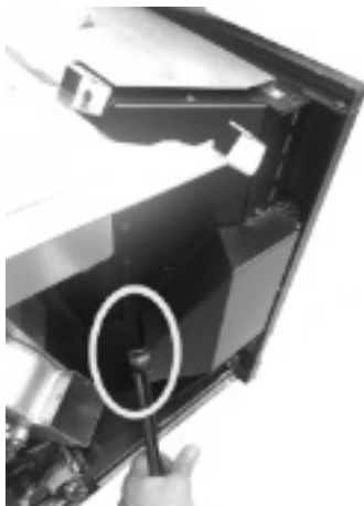
Fig. 41 - Rompa la esquina
