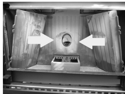
Fig. 111 - Extracción de las paredes laterales de hierro fundido
