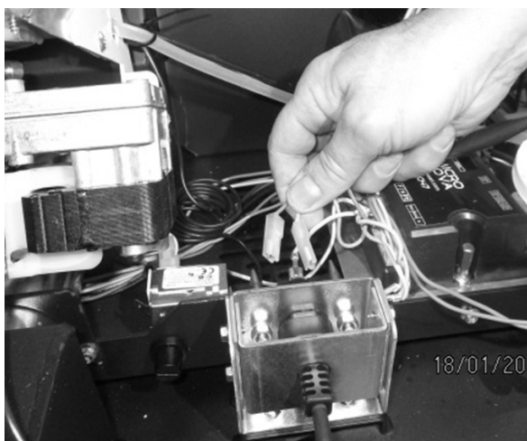
Fig. 88 - Desconexión del terminal faston (azul - marrón)
