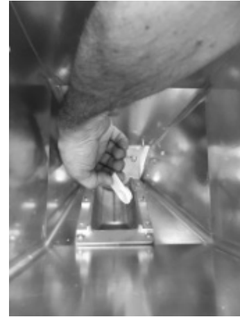
Fig. 95 - Extracción del cojinete
