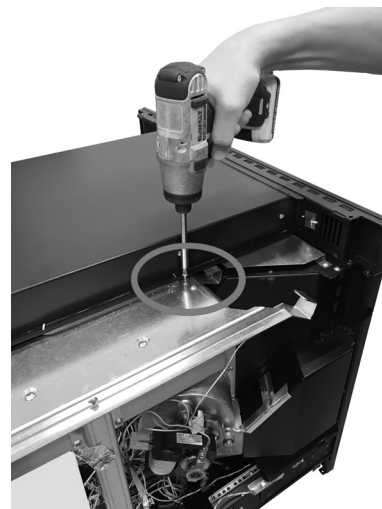
Fig. 58 - Fijación central del cajón
