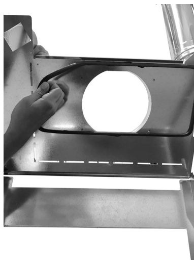
Fig. 54 - Extraiga la junta
