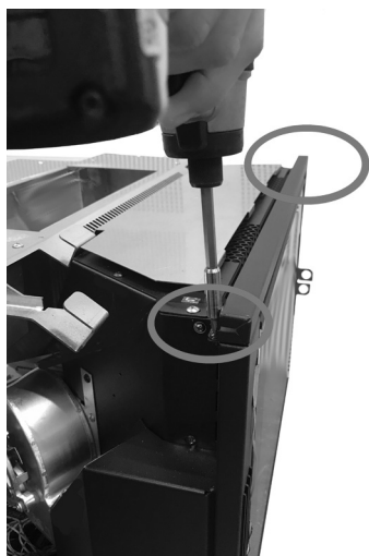
Fig. 53 - Extraiga el perfil superior
