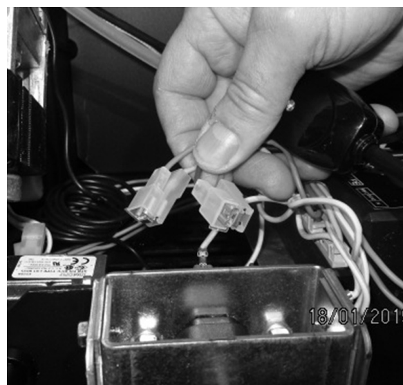
Fig. 89 - Conexión de los terminales faston dobles
