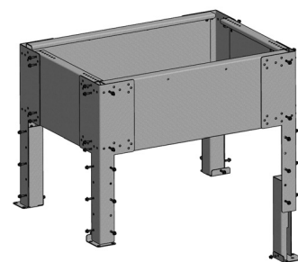
Fig. 37 - Monte las patas y el alargador
