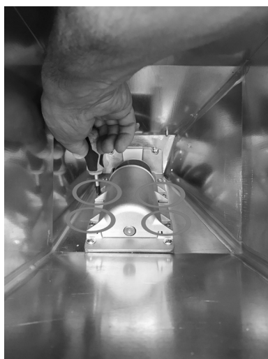
Fig. 91 - Extracción de los tornillos
