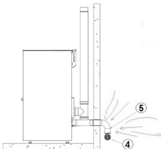
Fig. 3 - Toma de aire en caso de instalación estanca
