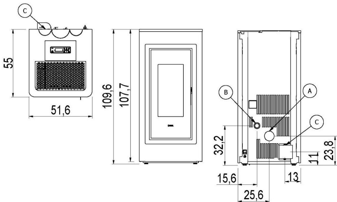
Fig. 8 - Dimensiones generales: Koba 11 - Koba Plus 11
