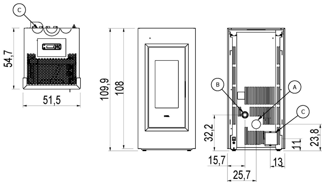
Fig. 7 - Dimensiones generales: Prince 11 - Prince Plus 11
