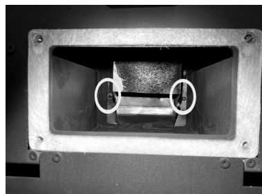
Fig. 82 - Desenrosque los tornillos
