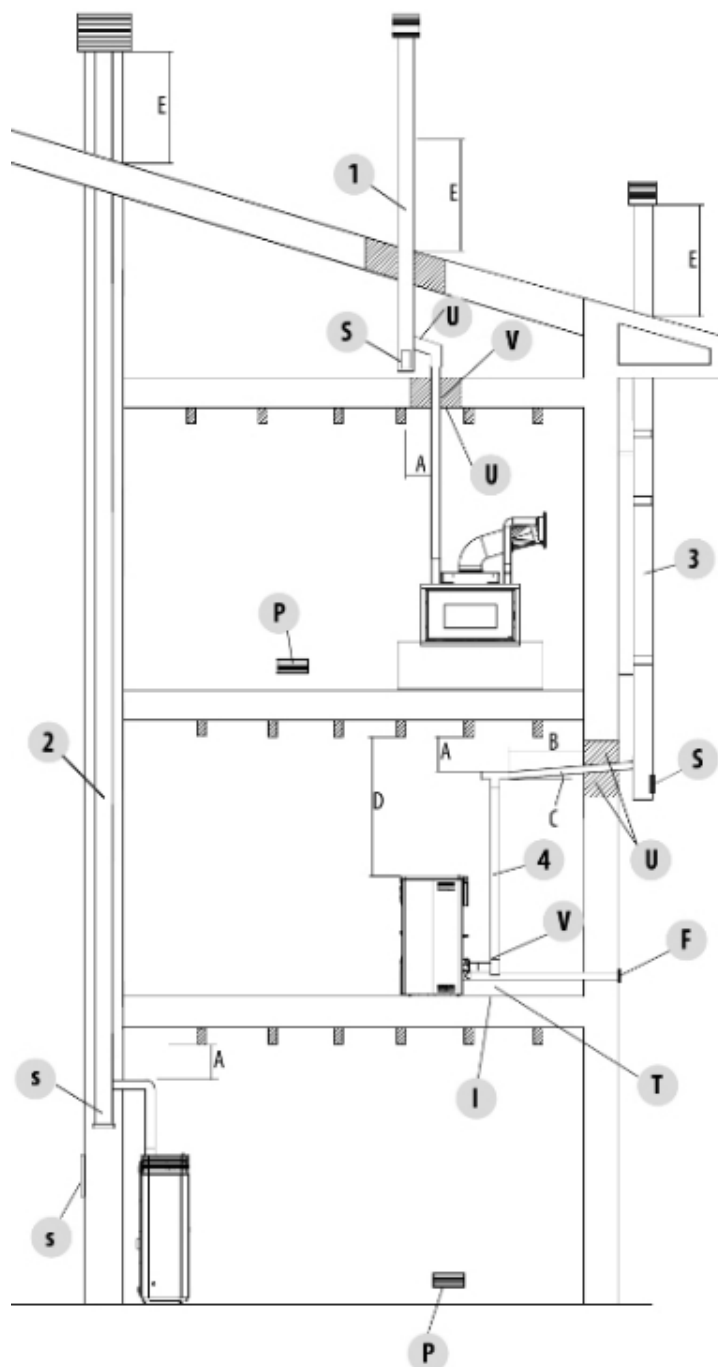
Fig. 5 - Sistema de evacuación de humos
