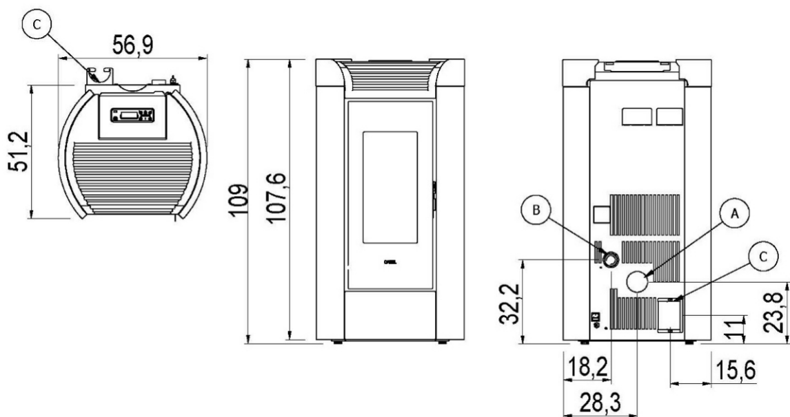
Fig. 9 - Dimensiones generales: Fenice 11 - Fenice Plus 11
