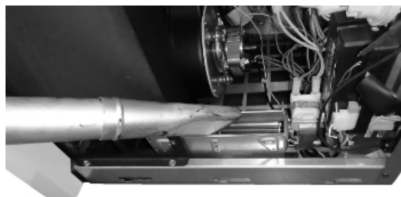
Fig. 86 - Limpieza ventilador ambiente
