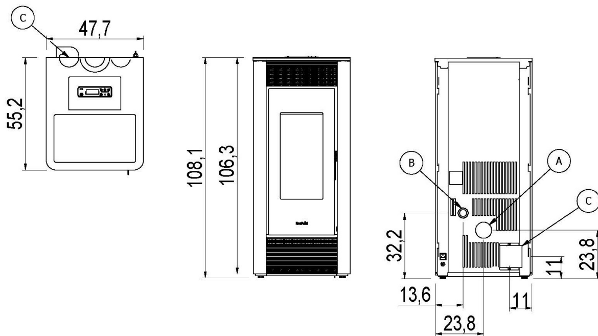
Fig. 10 - Dimensiones generales: Indaco 11
