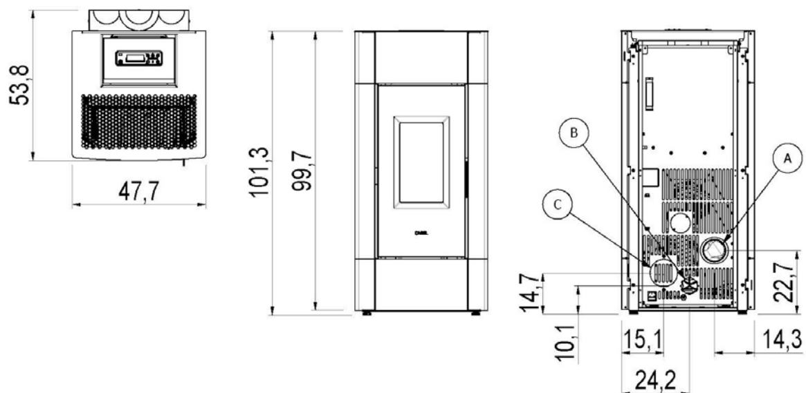
Fig. 18 - Dimensiones generales: Cristal Plus 9
