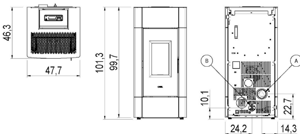
Fig. 17 - Dimensiones generales: Cristal 9
