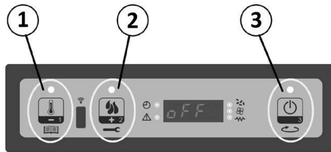
Fig. 72 - Display 3 tasti
