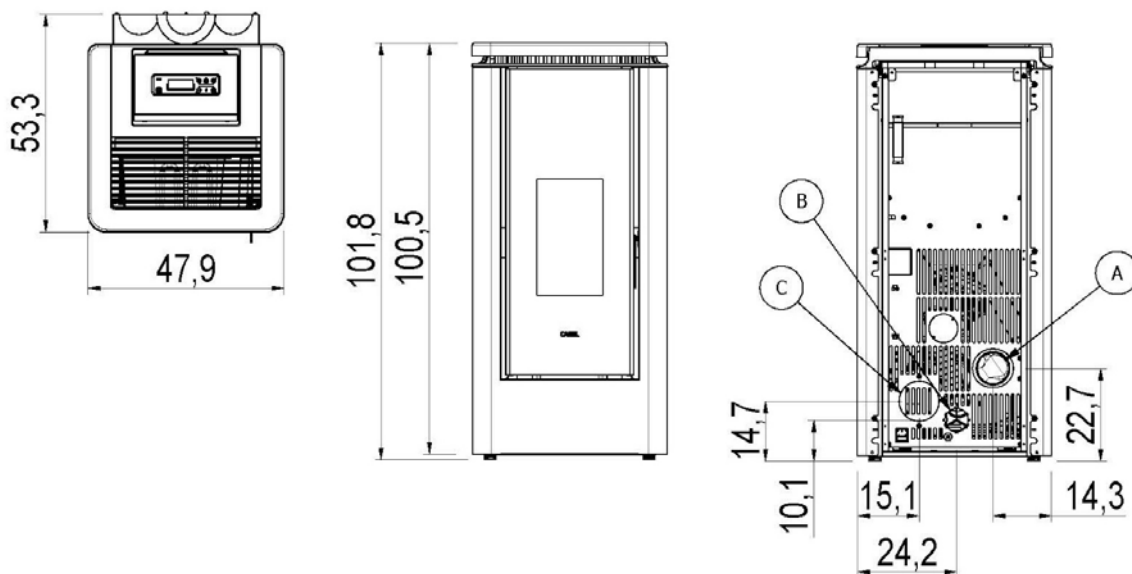
Fig. 19 - Dimensiones generales: Icon Plus 9
