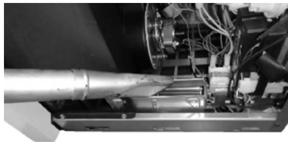
Fig. 83 - Limpieza ventilador ambiente (Mithos 3 Plus 12/14)
