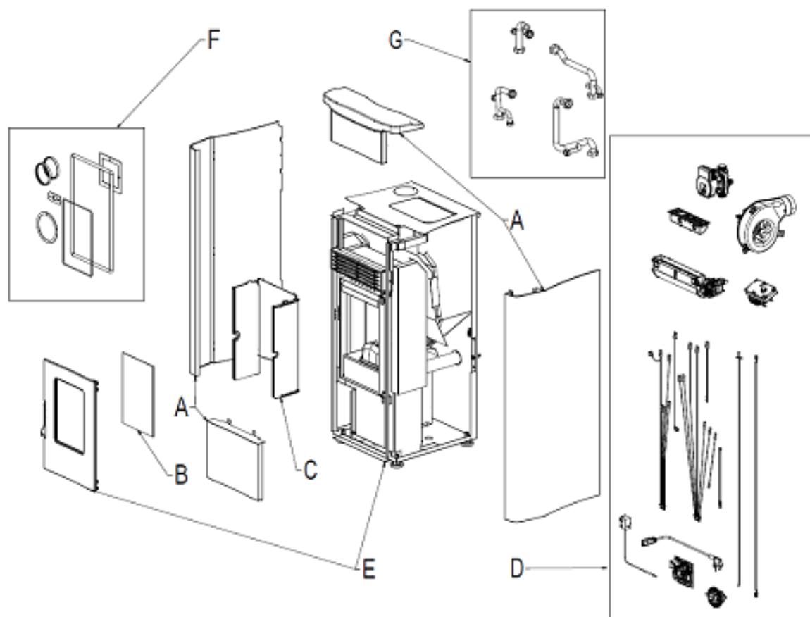
Fig. 1 - Dibujo explotado
