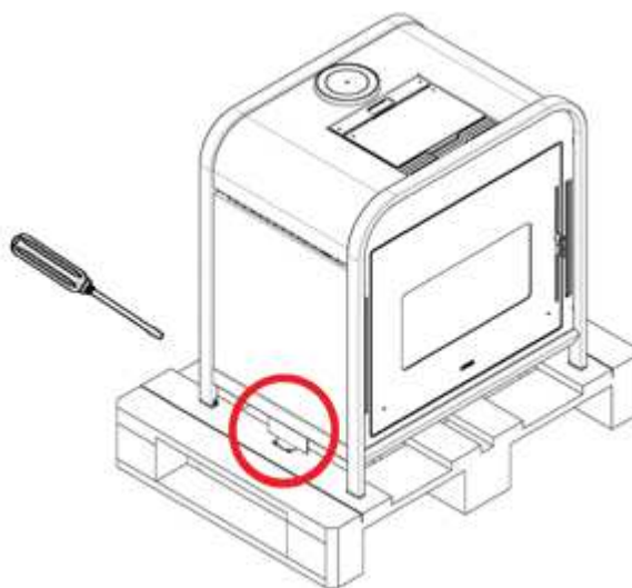
Fig. 1 - Extracción de los tornillos y de los estribos
