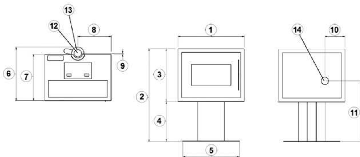
Fig. 16 - Dimensiones generales: QUASIMODO³ UP
