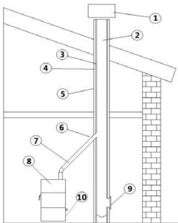
Fig. 2 - Componentes chimenea
