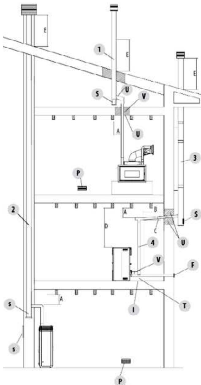
Fig. 12 - Sistema de evacuación de humos
