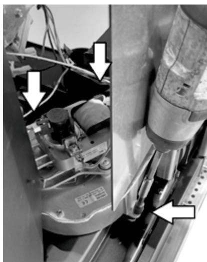
Fig. 63 - Quite los tornillos - Limpieza 1
