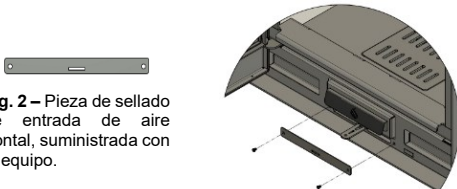
Fig. 3 – Retire los tornillos; coloque la pieza de sellado y vuelva a apretar los tornillos.
