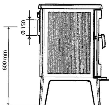
Conexión trasera
