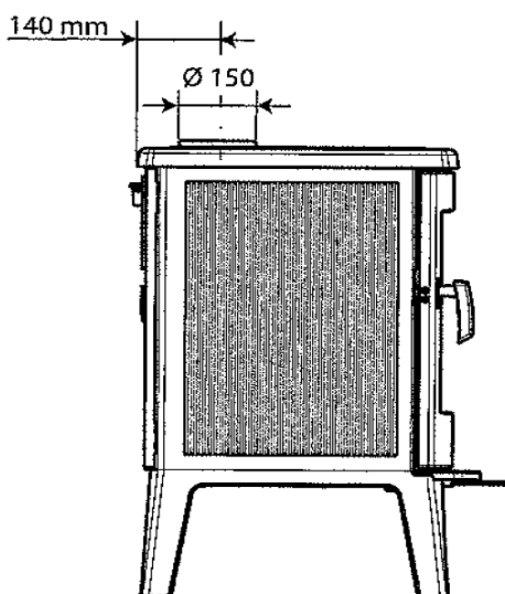
Conexión superior
