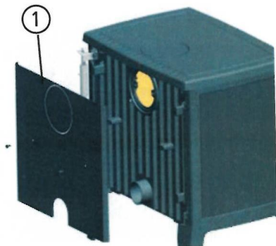
Fig 4.4 Desmontar la chapa posterior.
