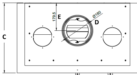
Vue supérieure
