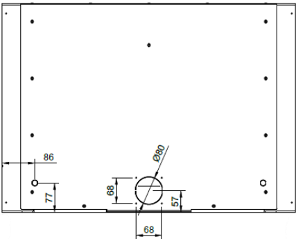
Vista inferior
