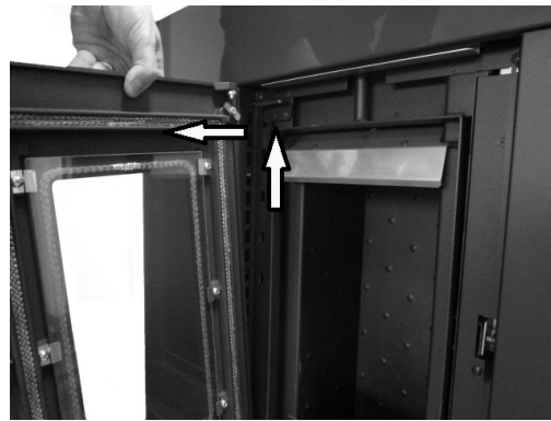
Fig. 26 - Desmontaje de la puerta
