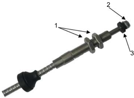
Fig. 47: Instalación de la unidad de control
