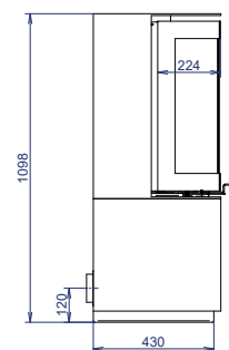
Zijaanzicht / Vue de côté Met woodbox / Avec niche à bois
