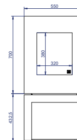
Vooraanzicht / Vue de face Met woodbox / Avec niche à bois
