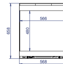
Vooraanzicht / Vue de face Zonder woodbox / Sans niche à bois
