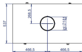
Bovenaanzicht / Vue de dessus
