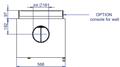
Bovenaanzicht / Vue de dessus
