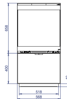
Vooraanzicht / Vue de face Met woodbox / Avec niche à bois
